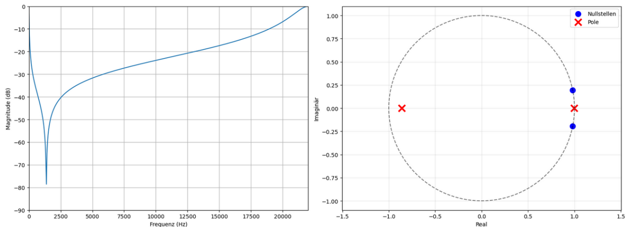
Abbildung 1: Frequenzgang und Pol- und Nullstellen von der Bandsperre
