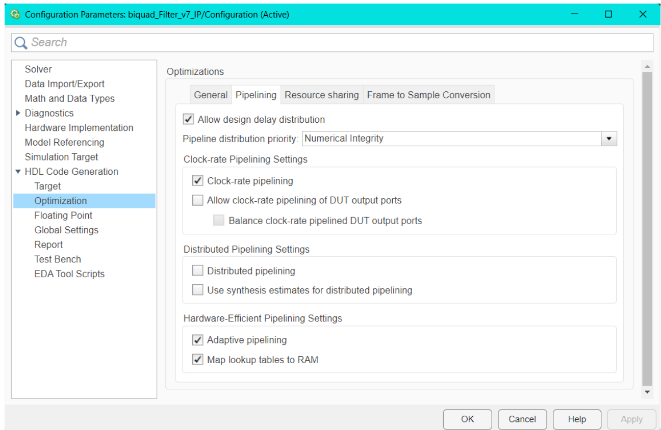
Abbildung 41.7.: HDL Workflow: HDL Options/ Optimization/ Pipelining
