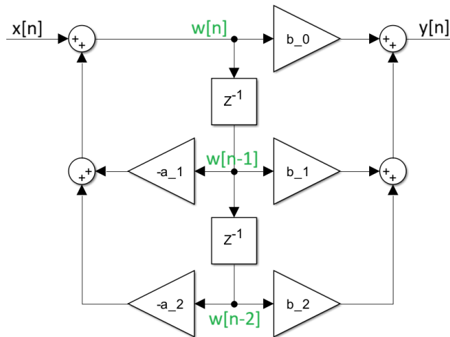
Abbildung 37.2.: Signalflussbild: Direktform 2
