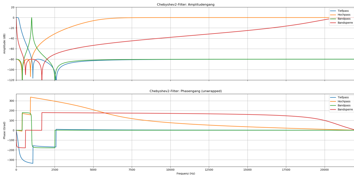
Abbildung 24.3.: Chebyshev2-Filter
