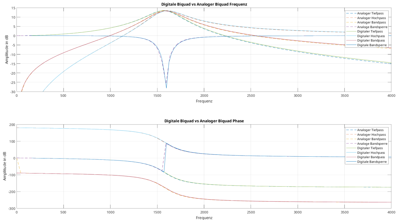
Abbildung 23.2.: Vergleich zwischen analogen und digitalen Frequenz- und Phasengang
