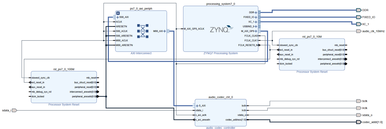
Abbildung 41.10.: Reference Design
