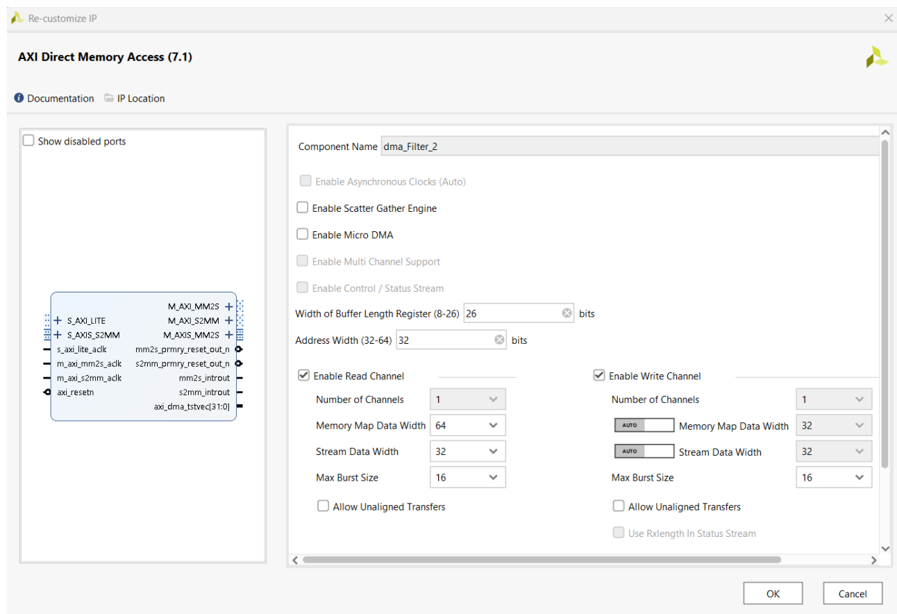
Abbildung 41.12.: AXI-DMA Config
