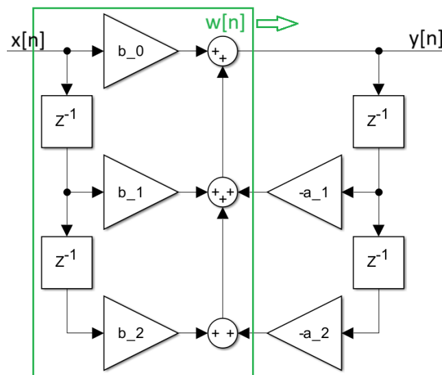
Abbildung 37.1.: Signalflussbild: Direktform 1
