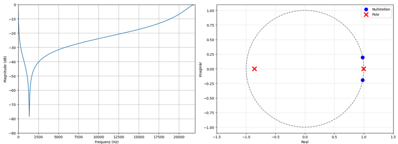
Abbildung 26.1.: Frequenzgang und Pol- und Nullstellen von der Bandsperre
