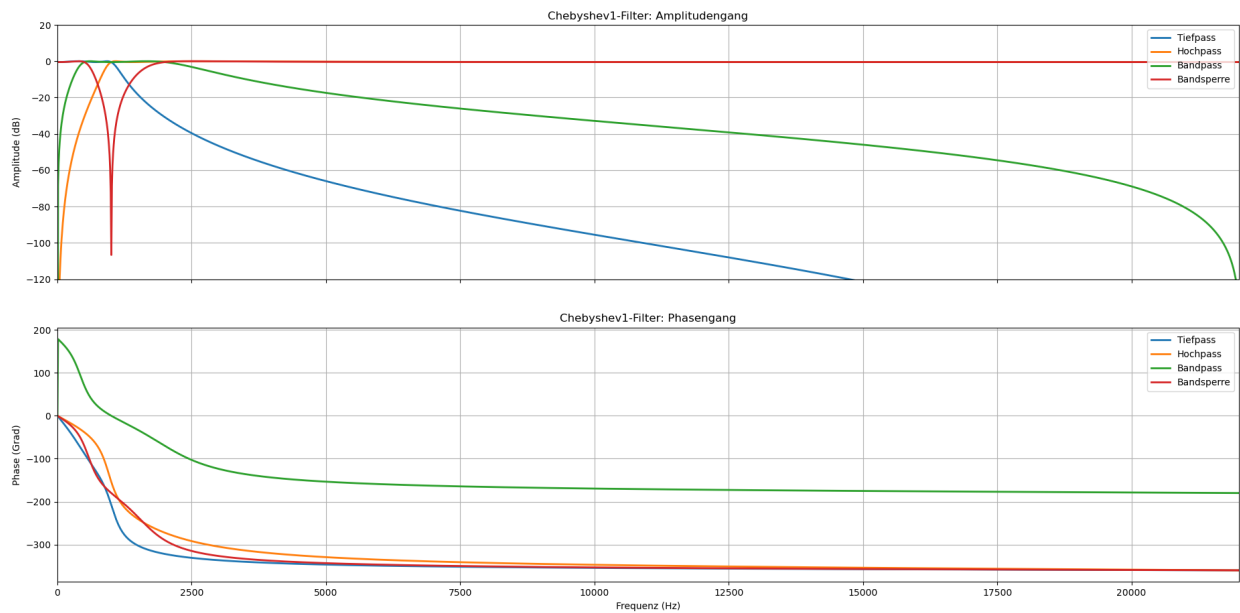
Abbildung 24.2.: Chebyshev1-Filter
