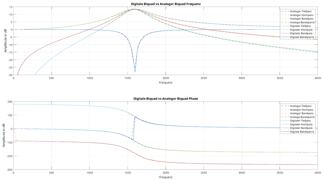
Abbildung 22.2.: Vergleich zwischen analogen und digitalen Frequenz- und Phasengang
