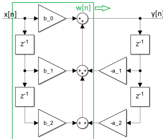
Abbildung 13.1.: Signalflussbild: Direktform 1
