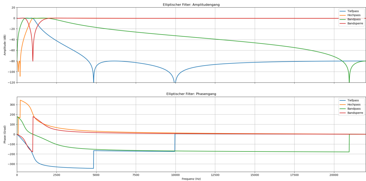
Abbildung 23.4.: Elliptischer Filter
