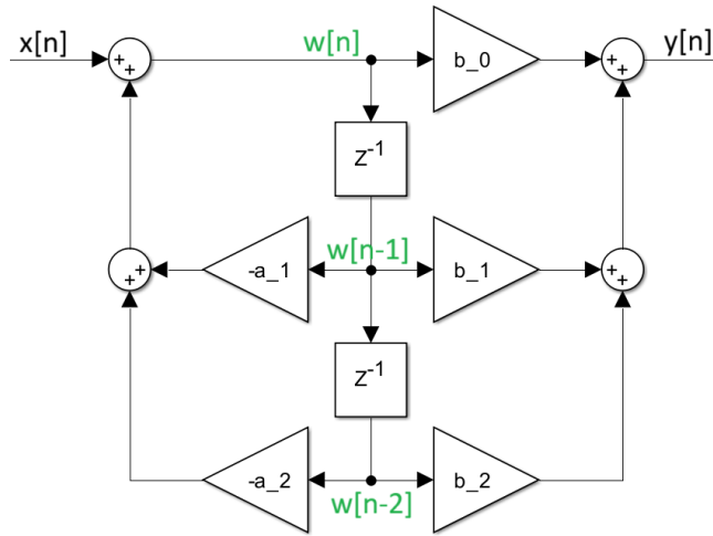
Abbildung 13.2.: Signalflussbild: Direktform 2
