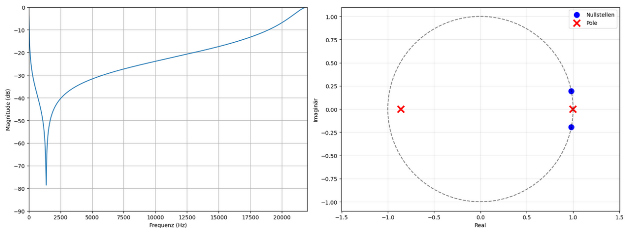
Abbildung 25.1.: Frequenzgang und Pol- und Nullstellen von der Bandsperre
