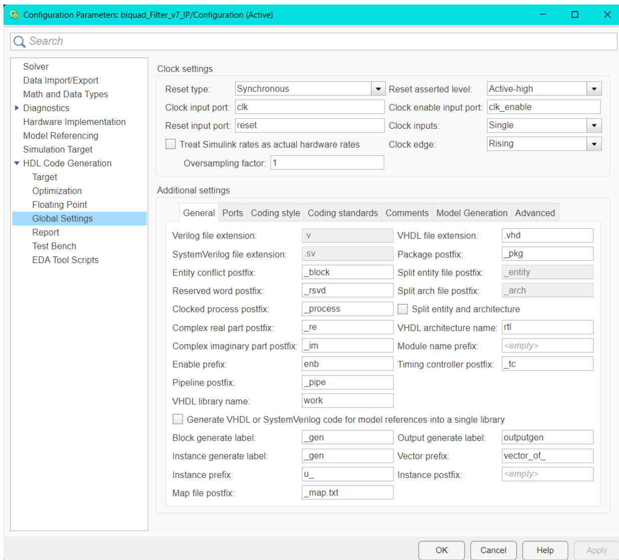
Abbildung 0.8: HDL Workflow: HDL Options/ Global Settings
