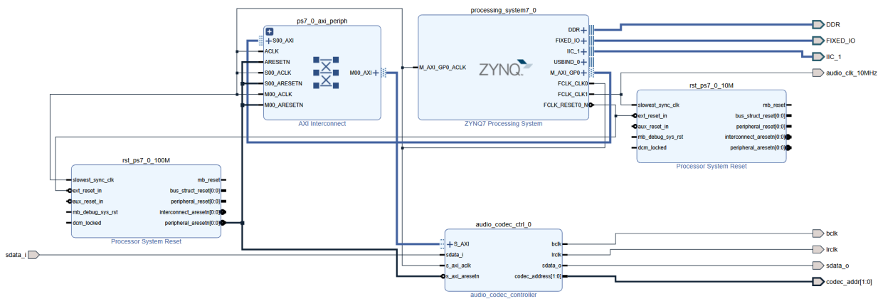
Abbildung 0.10: Reference Design
