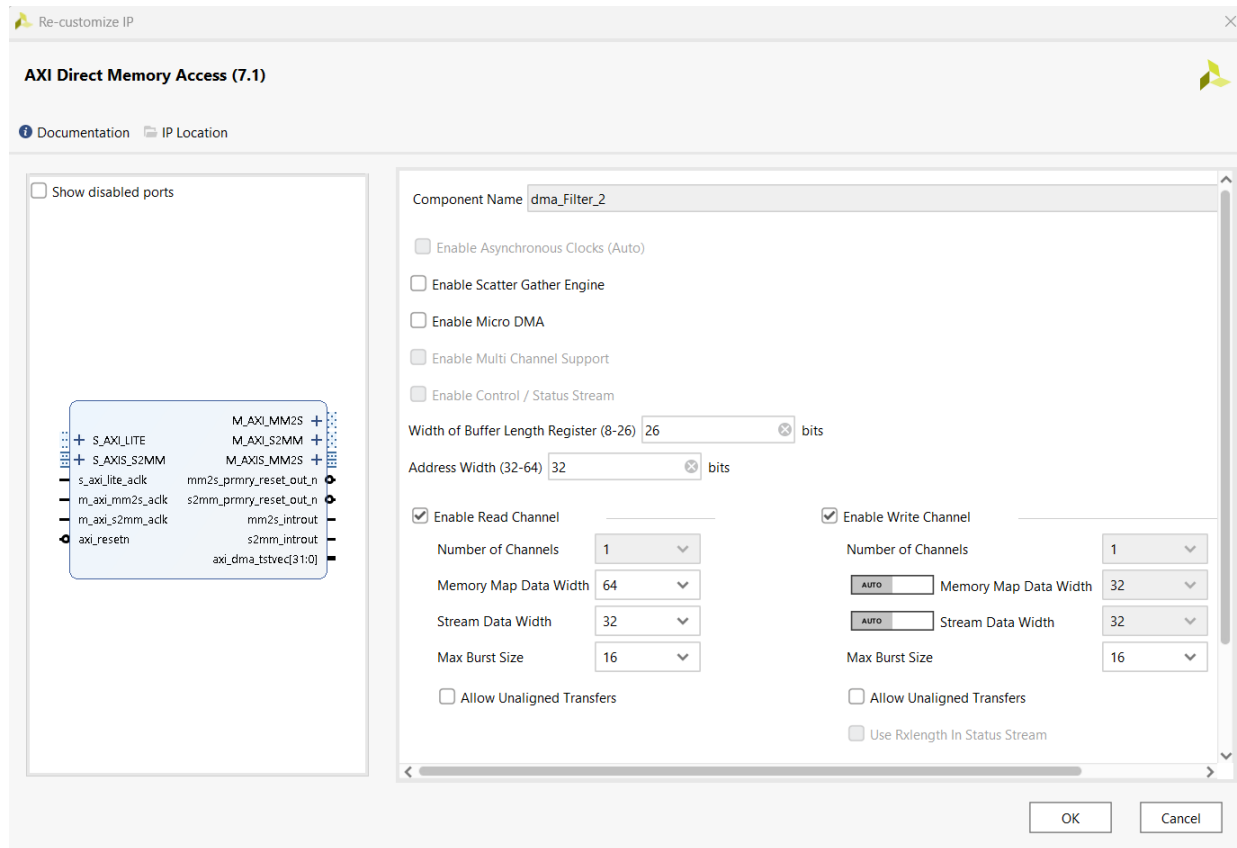
Abbildung 0.12: AXI-DMA Config
