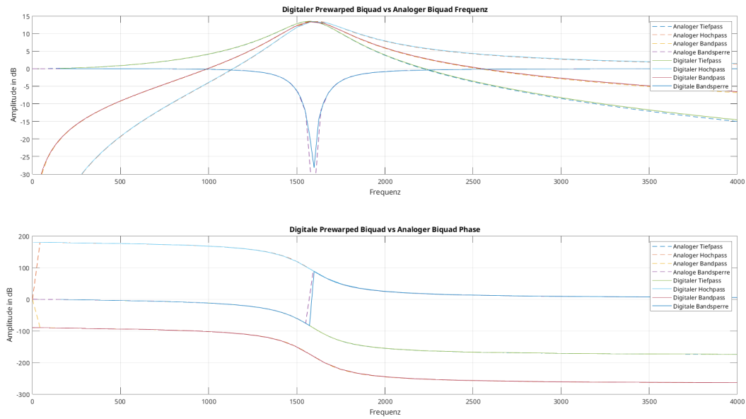
Abbildung 16.3.: Vergleich zwischen analogen und digitalen (Prewarped) Frequenz- und Phasengang
