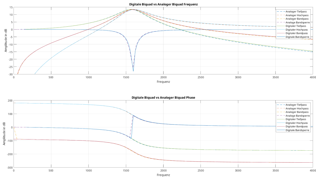
Abbildung 8.2.: Vergleich zwischen analogen und digitalen Frequenz- und Phasengang
