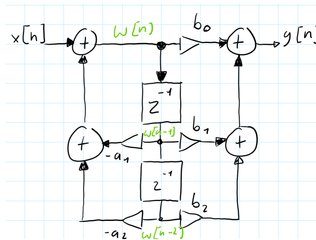
Abbildung 5.2.: Signalflussbild: Direktform 2
