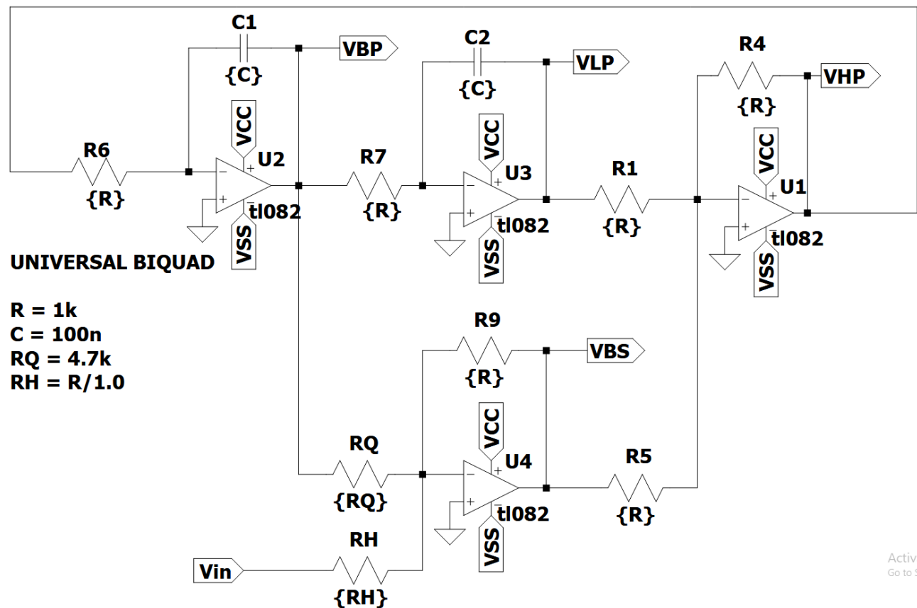
Abbildung 16.1.: Analoge Biquad Schaltung
