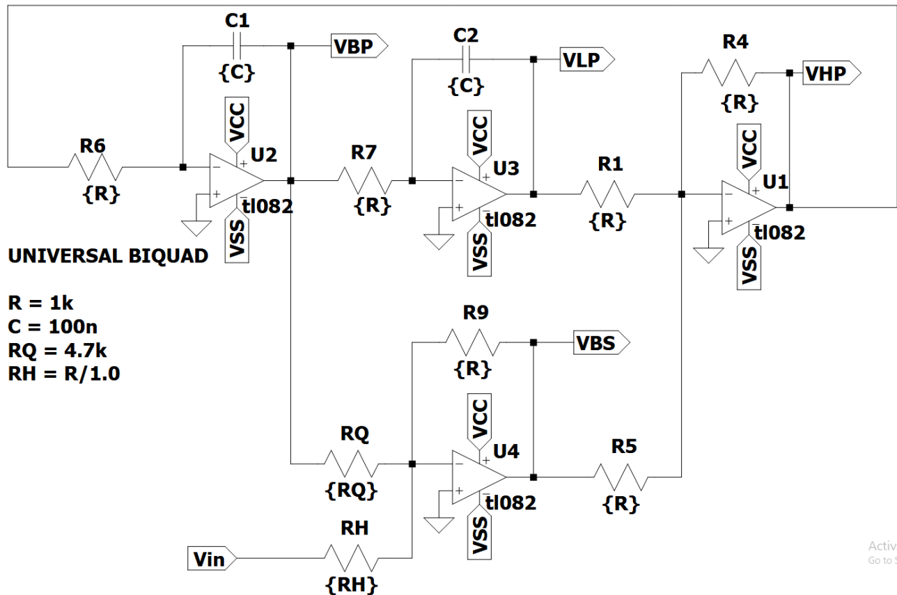
Abbildung 8.1.: Analoge Biquad Schaltung
