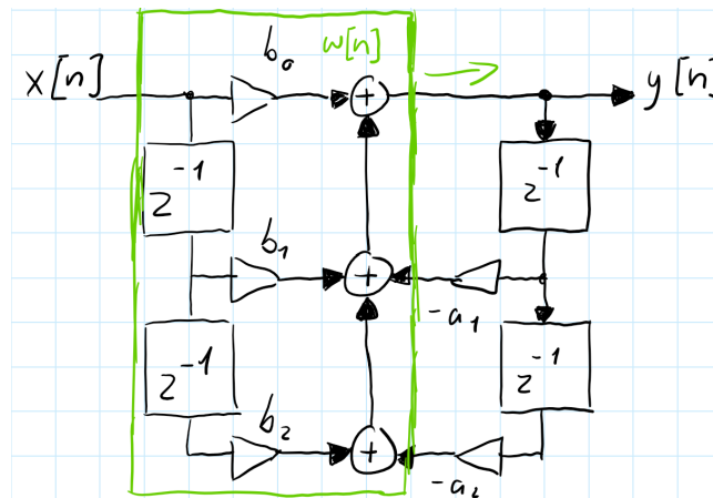
Abbildung 13.1.: Signalflussbild: Direktform 1
