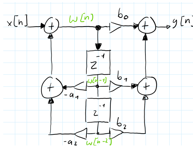
Abbildung 13.2.: Signalflussbild: Direktform 2
