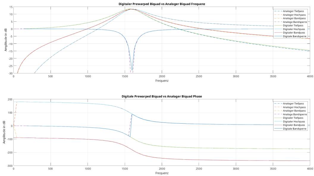
Abbildung 8.3.: Vergleich zwischen analogen und digitalen (Prewarped) Frequenz- und Phasengang
