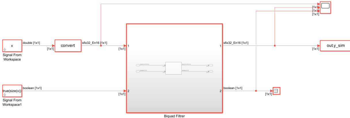
Abbildung 0.3: Simulink Filter
