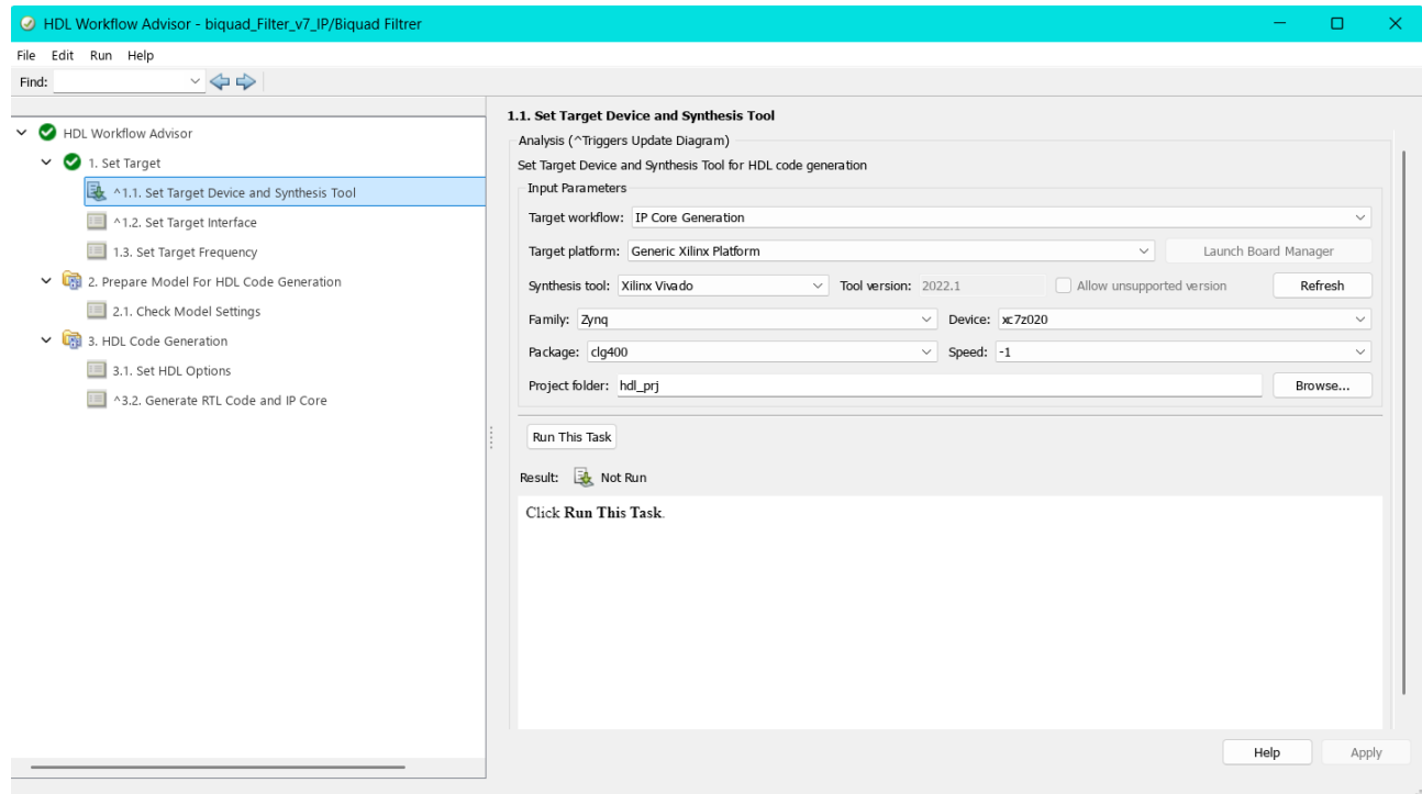
Abbildung 23.4.: HDL Workflow: Target Device
