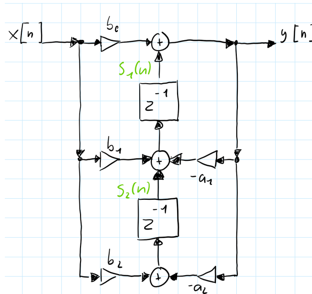
Abbildung 19.3.: Signalflussbild: Transponierte Direktform 2
