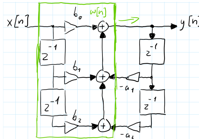
Abbildung 16.1.: Signalflussbild: Direktform 1
