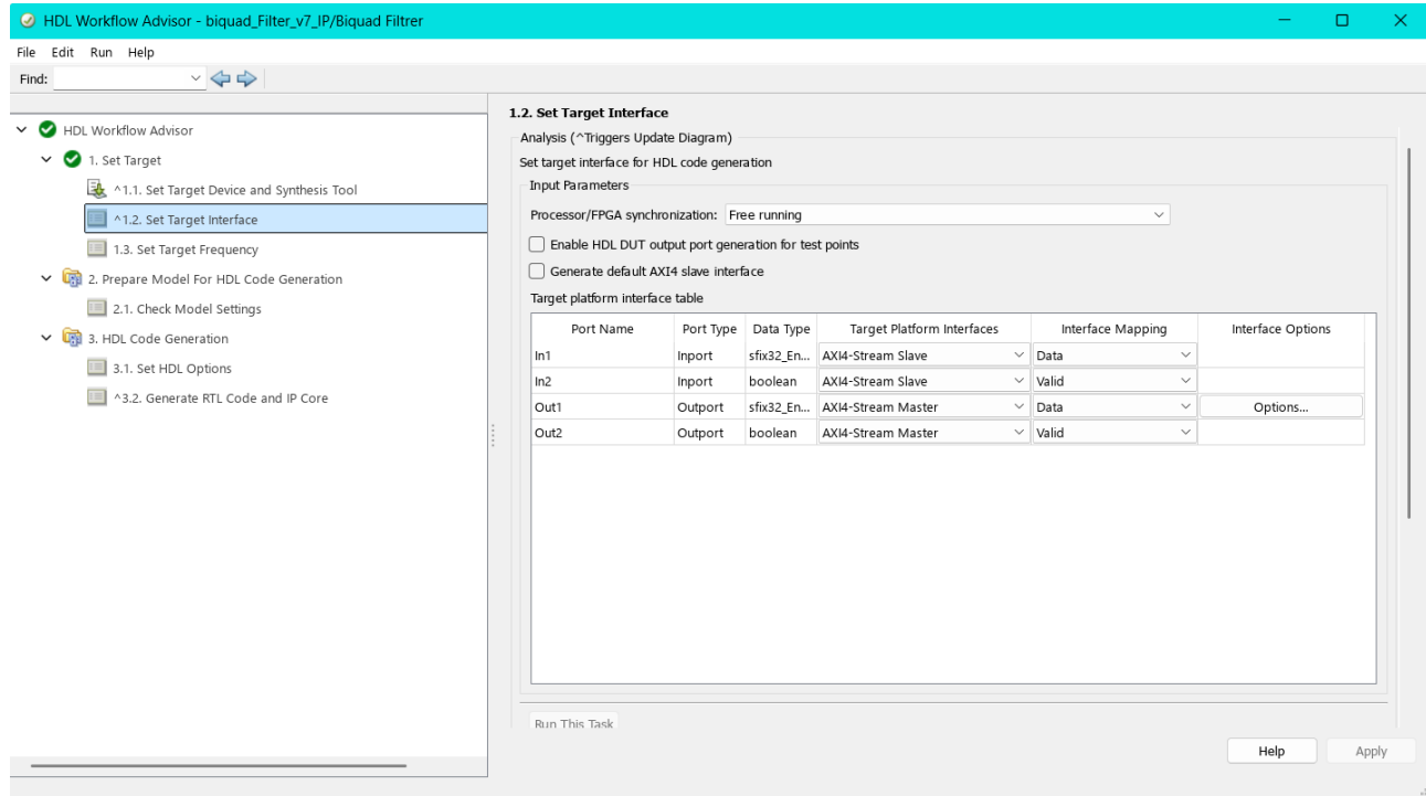
Abbildung 20.5.: HDL Workflow: Target Interface
