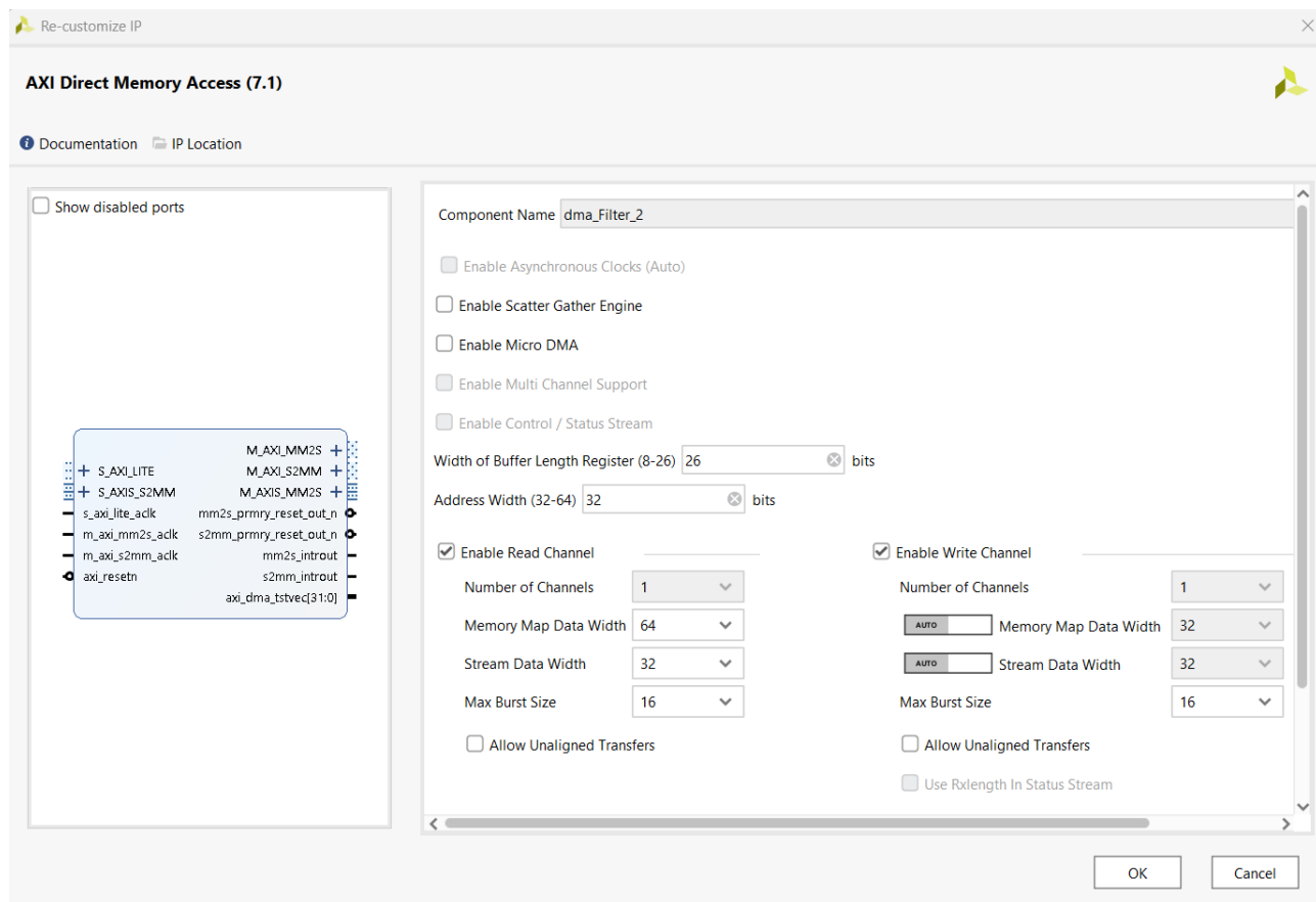
Abbildung 20.12.: AXI-DMA Config
