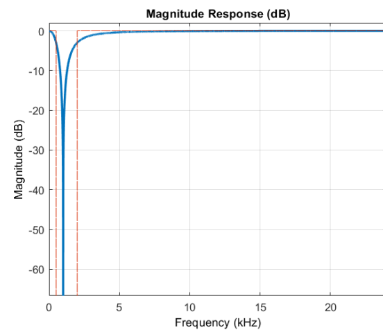
(b) Digitaler Butterworth-Bandstopfilter 2. Ordnung
