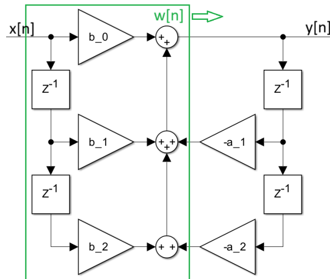
Abbildung 32.1.: Signalflussbild: Direktform 1
