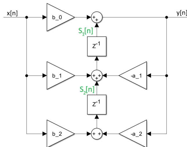
Abbildung 18.3.: Signalflussbild: Transponierte Direktform 2
