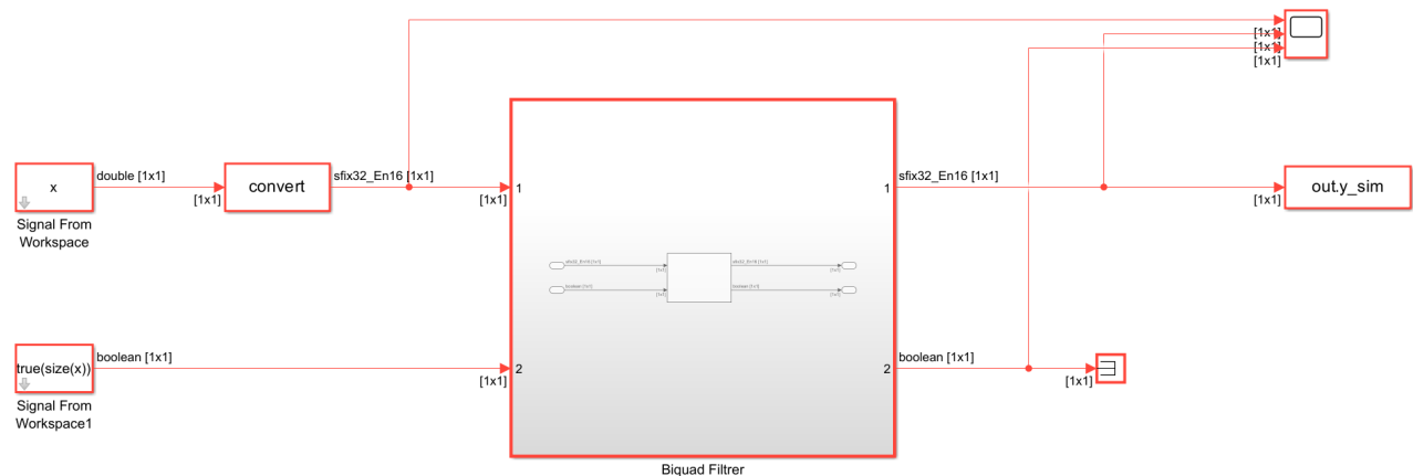
Abbildung 22.3.: Simulink Filter
