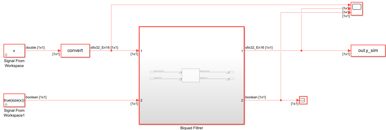
Abbildung 41.3.: Simulink Filter
