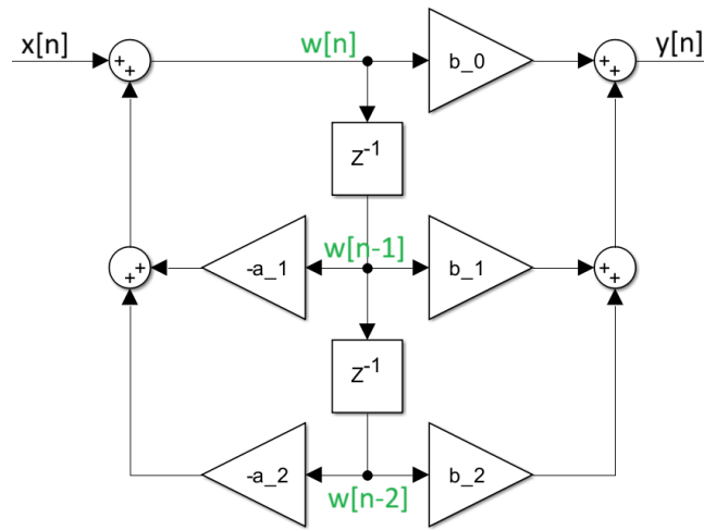
Abbildung 20.2.: Signalflussbild: Direktform 2
