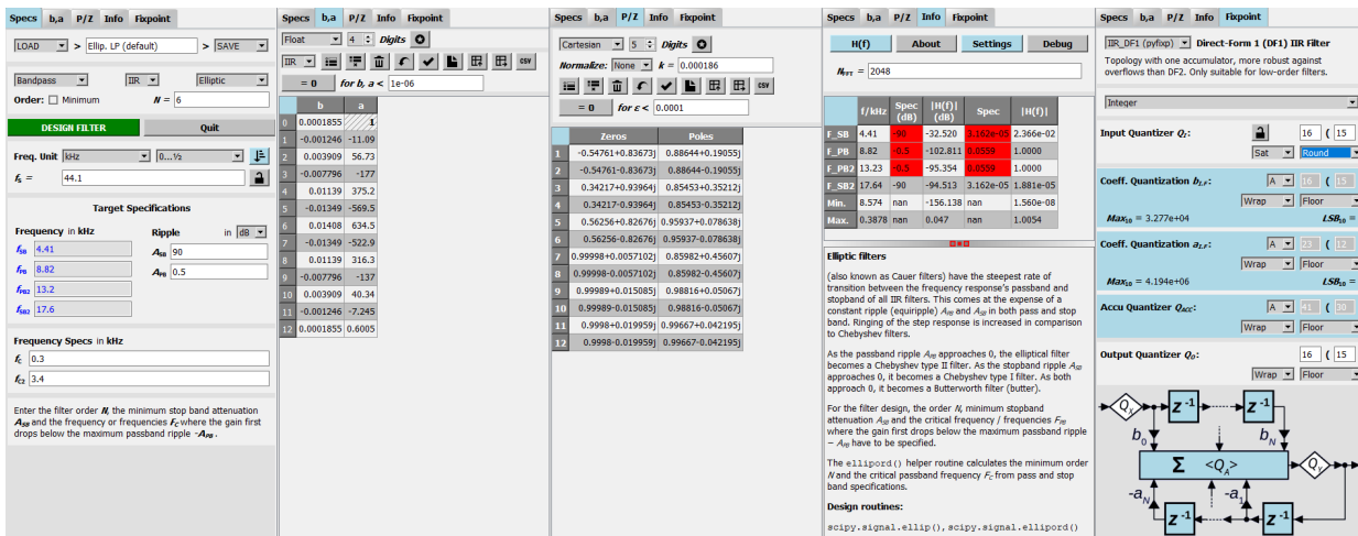
Abbildung 0.1: Pyfda: Entwurfsparameter
