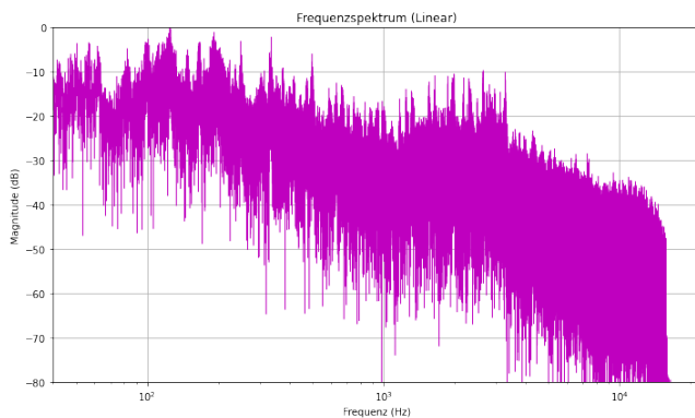
(a) Frequenzspektrum vor dem Filtern
