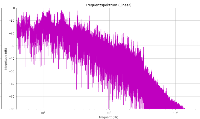
(b) Frequenzspektrum nach der Tiefpassfilterung
