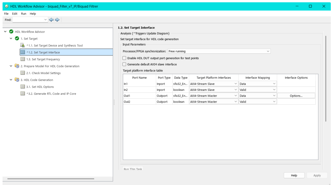
Abbildung 25.5.: HDL Workflow: Target Interface
