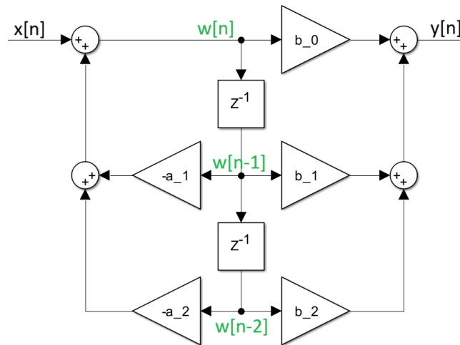
Abbildung 20.2.: Signalflussbild: Direktform 2
