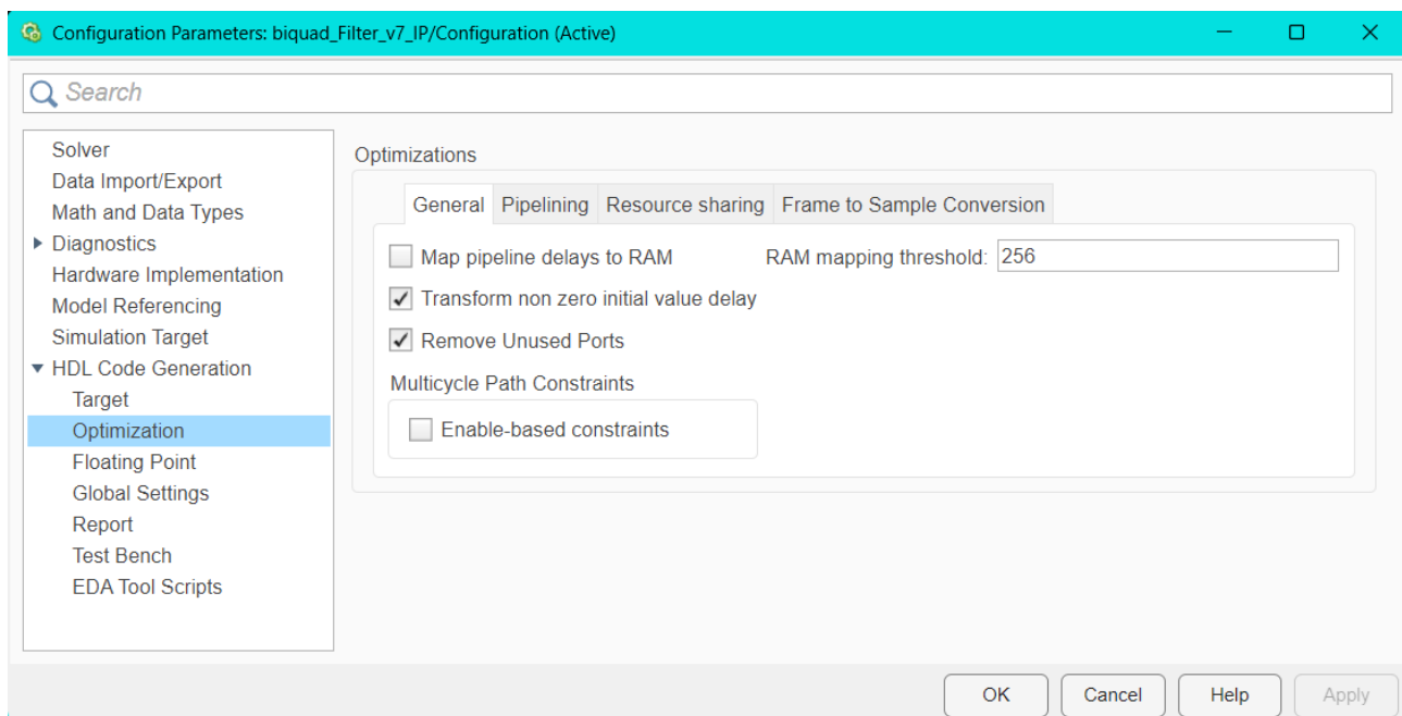
Abbildung 25.6.: HDL Workflow: HDL Options/ Optimization/ General
