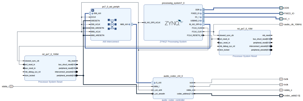
Abbildung 23.10.: Reference Design
