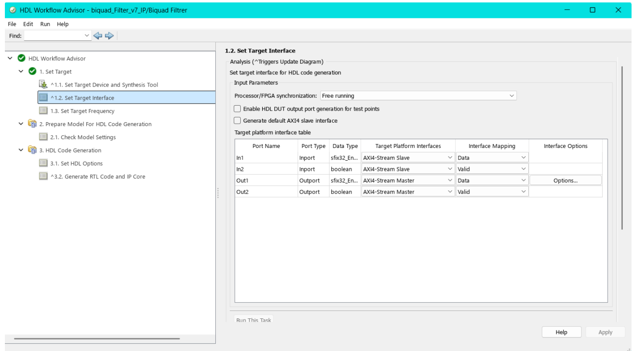
Abbildung 23.5.: HDL Workflow: Target Interface
