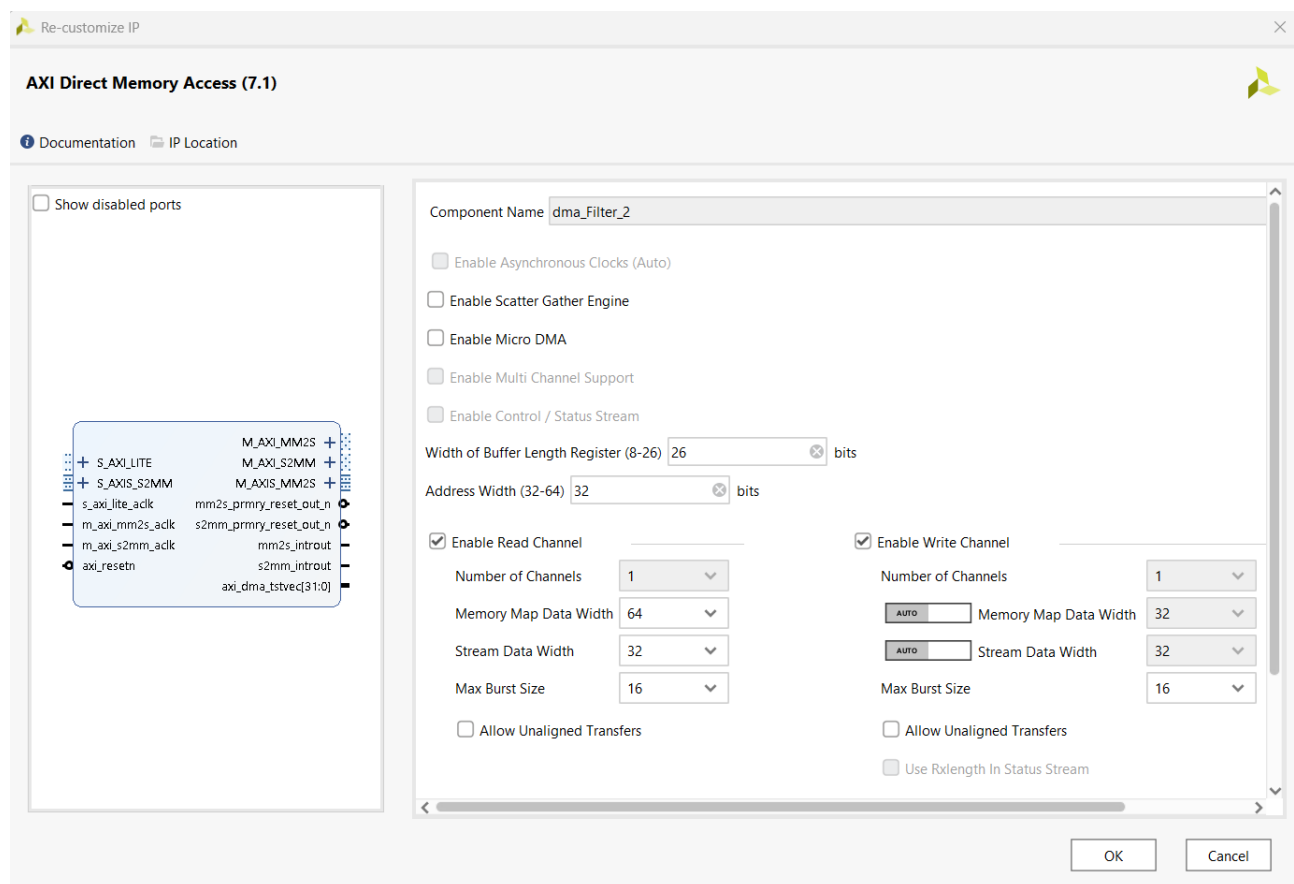
Abbildung 23.12.: AXI-DMA Config
