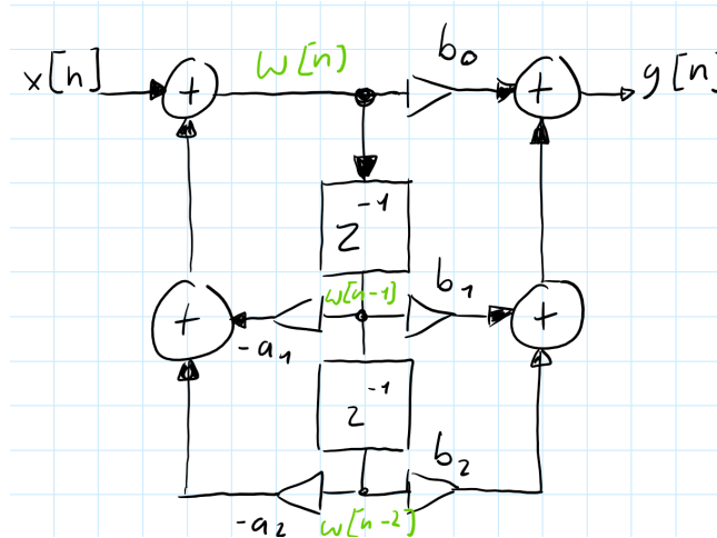
Abbildung 19.2.: Signalflussbild: Direktform 2
