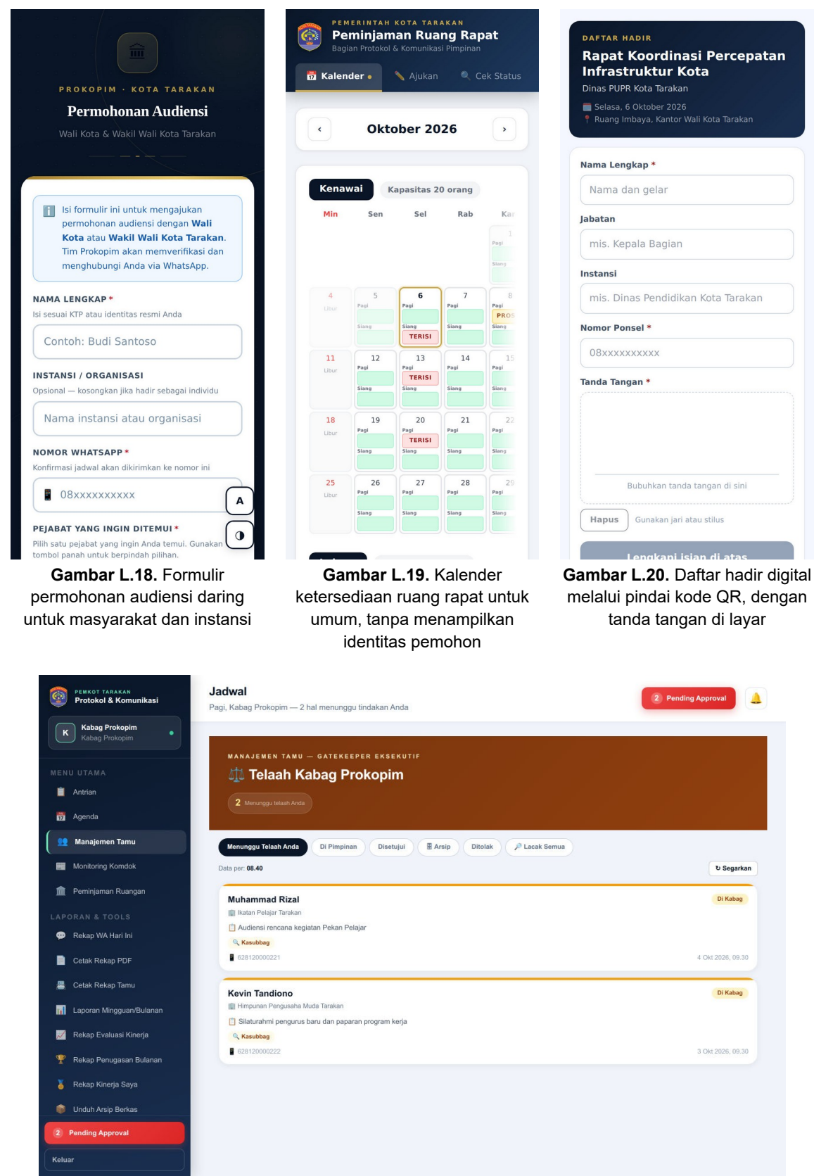
Gambar L.21. Manajemen tamu: telaah berjenjang permohonan audiensi sampai menjadi agenda Pimpinan
