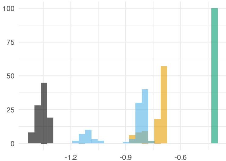
Vowel
