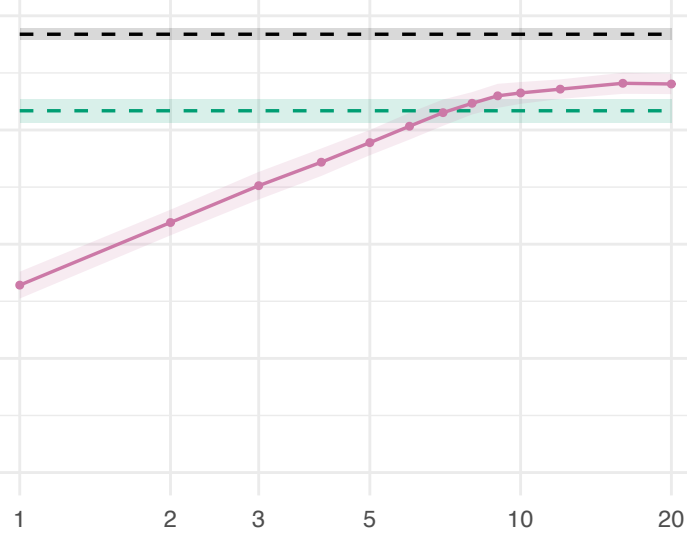
Vowel
