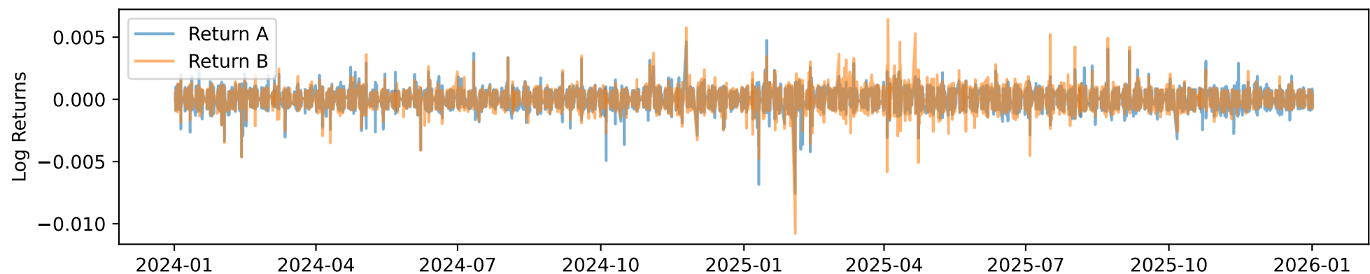
Asset Returns
