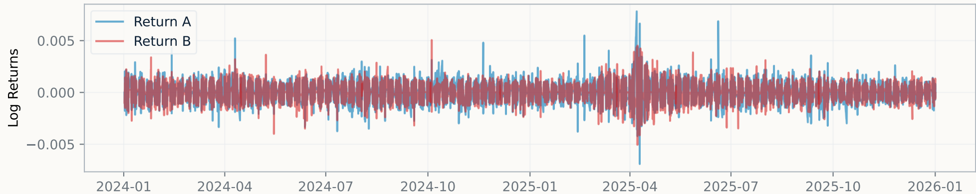
Asset Returns
