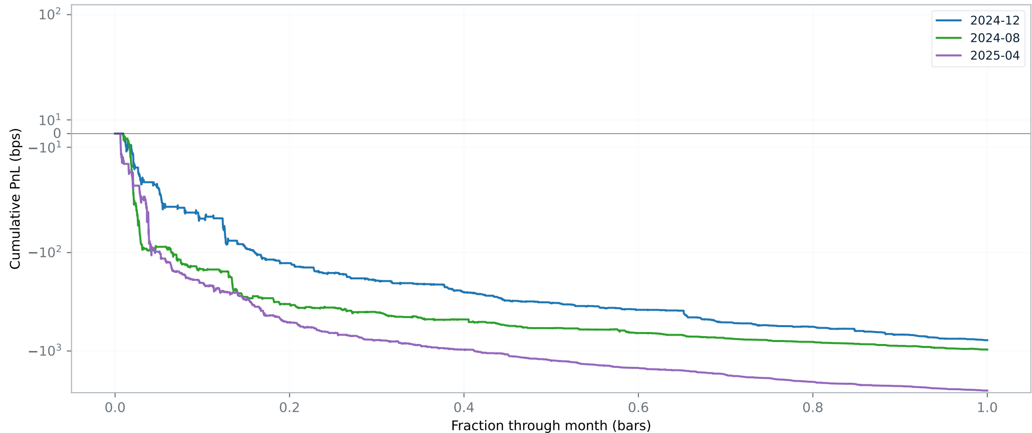
AUDUSD/NZDUSD — (2) Baseline — symlog y
