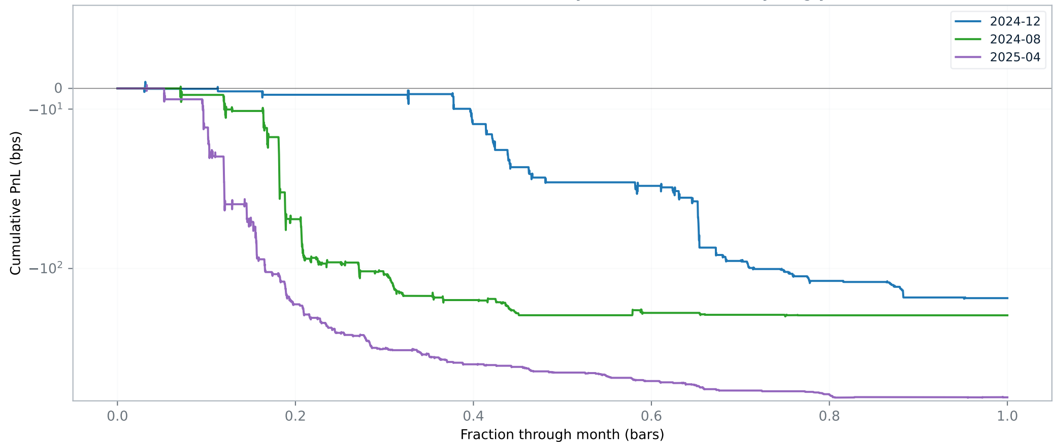
AUDUSD/NZDUSD — (4) MS-AR (dynamic threshold) — symlog y
