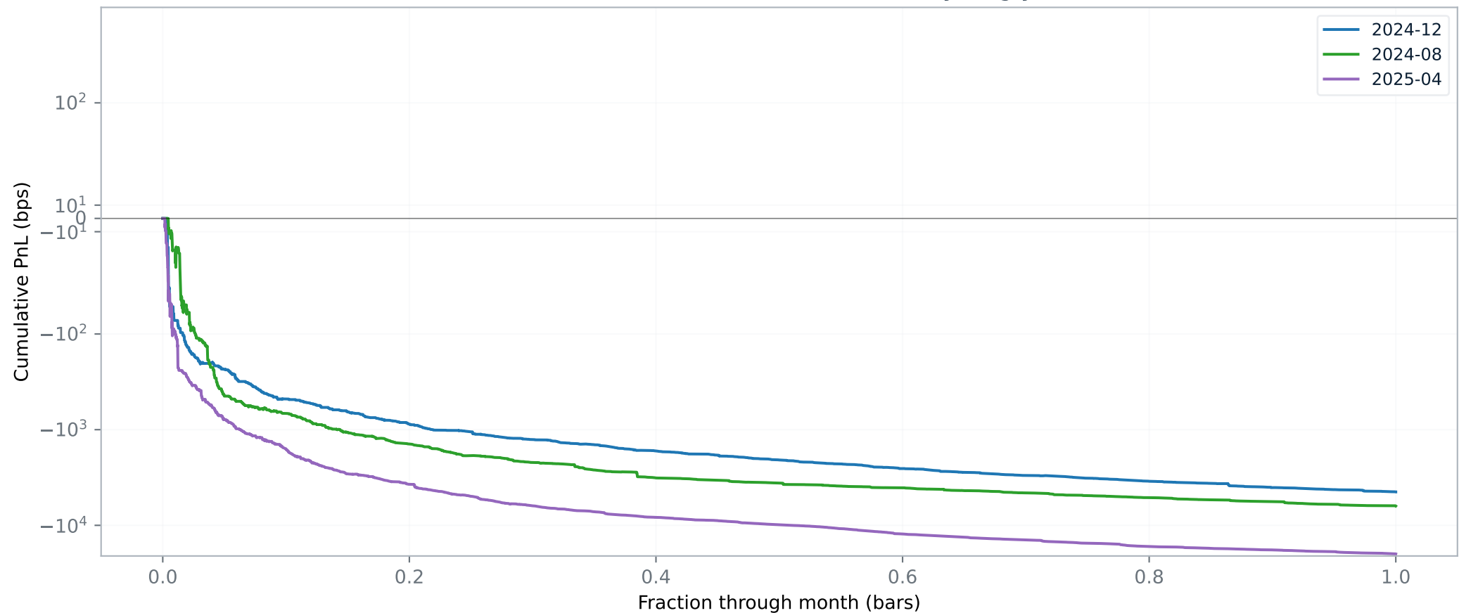
EURNOK/EURSEK — (2) Baseline — symlog y
