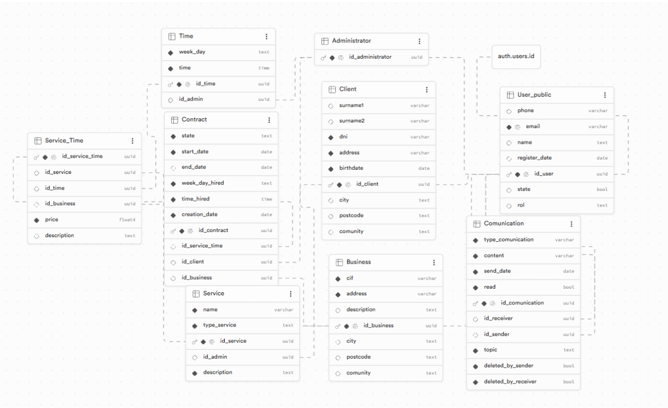
Ilustración 21: Esquema Public Supabase.
