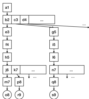
図 5.1 探索木
