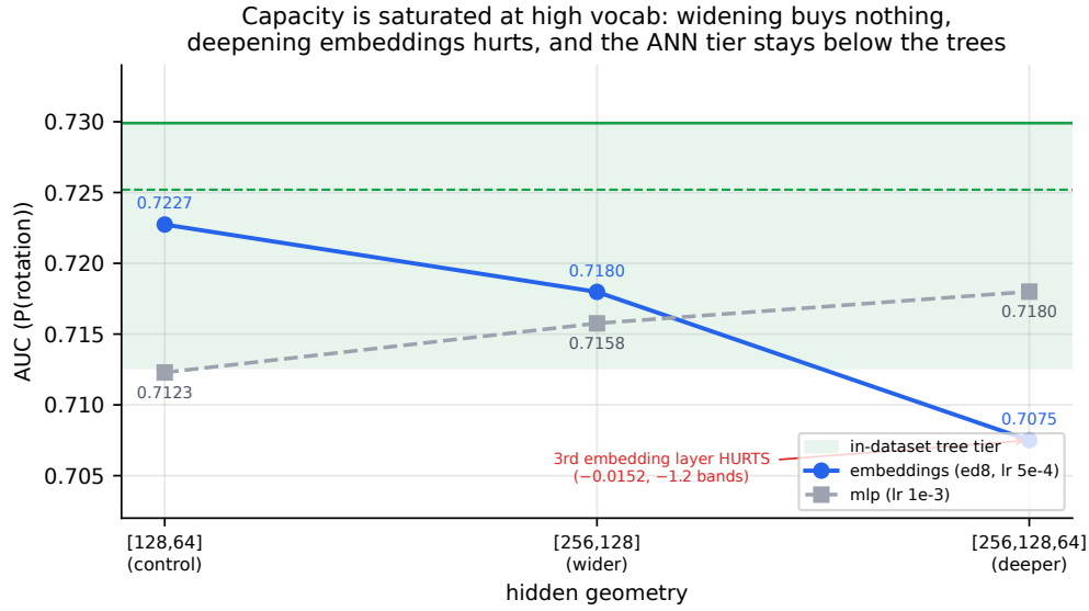
Figura 15: La capacidad es una palanca agotada para la red densa en vocabulario alto. Manteniendo lr en el mejor de cada topología y escalonando la geometría oculta [128,64] \rightarrow [256,128] \rightarrow [256,128,64] , ni la escalera embeddings (azul) ni la mlp (gris) supera su propio control por una banda; una tercera capa embeddings perjudica por 0,0152 ( \sim 1.2 bandas, el único movimiento fuera de banda), porque la profundidad extra diluye una entrada de embedding de entidad aprendida ya peor condicionada. El mejor mlp cierra a menos de +0,0047 del mejor embeddings , así que las dos familias empatan dentro de una banda — la capacidad, no el mecanismo de embeddings, fue la palanca — y todo el nivel ANN se mantiene \sim 0.2\text{--}0.6 banda bajo el nivel de los árboles dentro del dataset (sombreado, catboost 0,7252 hasta xgboost 0,7299).
