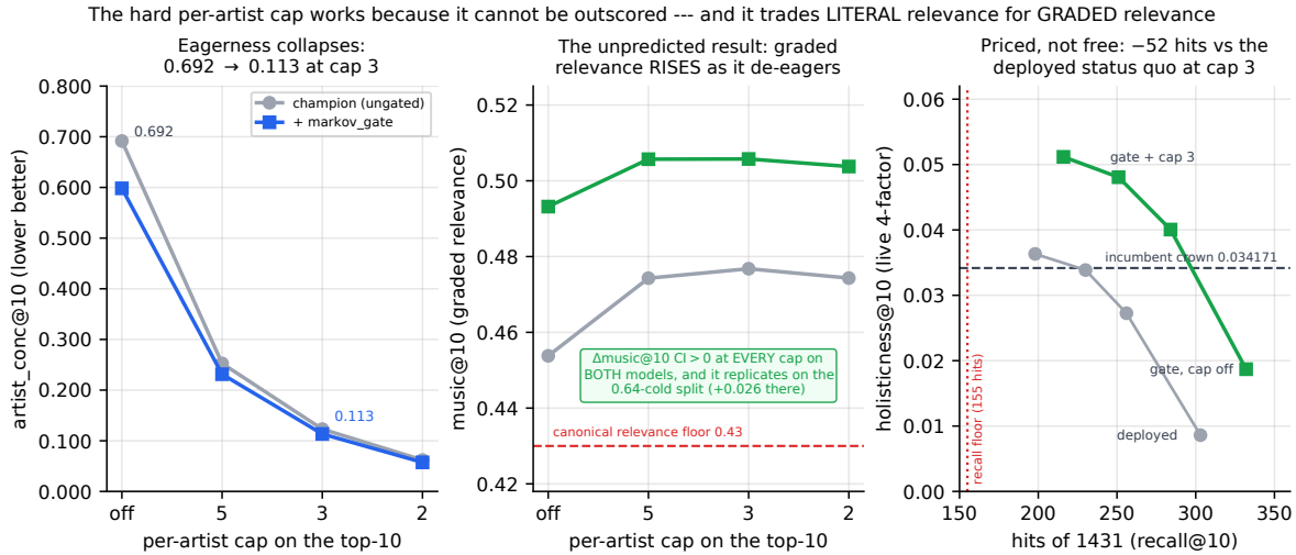
Figura 33: Izquierda: la concentración de artista se derrumba, 0,692→0,113 con tope 3 en el campeón con compuerta. Centro: el resultado que no se predijo — la relevancia graduada sube , con el IC pareado sobre cero en todos los topes y en ambos modelos, y se replica en la partición disjunta con 64% de fríos con +0,026. La preocupación pre-registrada era que un tope des-eagerizara degenerando en relleno genérico; ocurre lo contrario, porque los ítems promovidos desde el puesto 75 en adelante son más aptos musicalmente para la continuación real que las pistas del mismo artista que desplazan. Derecha: el precio, en el plano recall × corona. El tope tiene precio , no es gratis: compuerta + tope 3 cuesta 52 de 1431 aciertos exactos frente al statu quo desplegado, mientras aterrizas una holisticness@10 de generación 3 en torno al 40% por encima de la corona incumbente con 1,5× su recall. Todas las ramas superan el umbral de 155 aciertos, así que ninguna es una instancia de la patología de «maximizar holisticness prediciendo peor».
