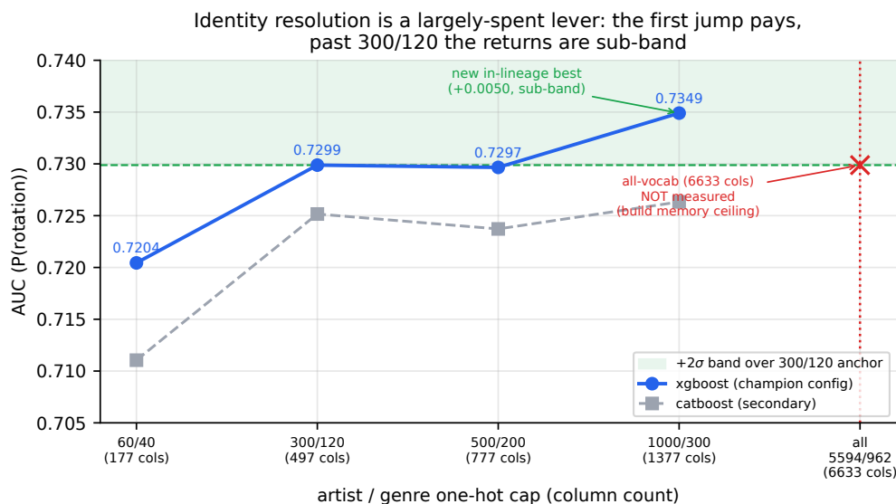
Figura 13: La palanca de resolución de identidad está en gran medida agotada. Manteniendo la config campeona congelada y moviendo solo el tope de one-hots de artista/género, la curva tope \rightarrow AUC sube abruptamente en el primer salto (60/40 \rightarrow 300/120, +0,75 banda) y luego se estanca : 300 \rightarrow 500 es plano ( -0,00022 , dentro del ruido) y 500 \rightarrow 1000 recupera solo +0,42 banda, así que la nueva mejor de linaje single-split (0,73490 en 1000/300) supera el ancla 300/120 por solo +0,00502 ( \sim 0.40 banda, dentro del sobre sombreado +2\sigma y por tanto una mejora sub-banda ). catboost (discontinua) sigue a xgboost en cada tope, \sim 0.005 – 0.009 por debajo — el manejo categórico nativo no compra ventaja de alta cardinalidad. El punto de vocabulario completo (6633 cols, \times rojo) está no medido : su build chocó con un techo de memoria del host en ambos intentos, un fallo de infraestructura más que un resultado de modelado.
