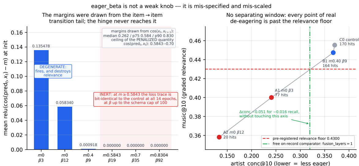
Figura 32: Izquierda: el resultado central de la campaña. La penalización realizada del hinge en la inicialización, reconstruida a partir de la inflación de la pérdida en la época 1 con inicialización compartida (semilla idéntica, así que inicialización y orden de lotes idénticos). Los márgenes se calibraron desde el coseno de transición ítem → ítem (mediana 0,262, p75 0,584, p90 0,830), pero la penalización actúa sobre predicción → actual , cuyo techo a lo largo del entrenamiento se sitúa entre 0,5843 y 0,70: con m \geq 0,5843 la cantidad penalizada nunca entra en el soporte del hinge y la traza de pérdida es idéntica bit a bit a la del control en las 14 épocas, con \beta hasta el tope del esquema. Derecha: donde el mando sí dispara, eagerness y relevancia son el mismo mecanismo. Empujar la predicción lejos del latente de la pista actual la empuja también fuera de la región donde vive la verdadera pista siguiente, así que no hay ventana entre un des-eagerness real y romper el umbral de relevancia. La línea de trazo y punto marca el comparador gratuito ya registrado que ninguna rama de aquí igualó dentro del umbral.
