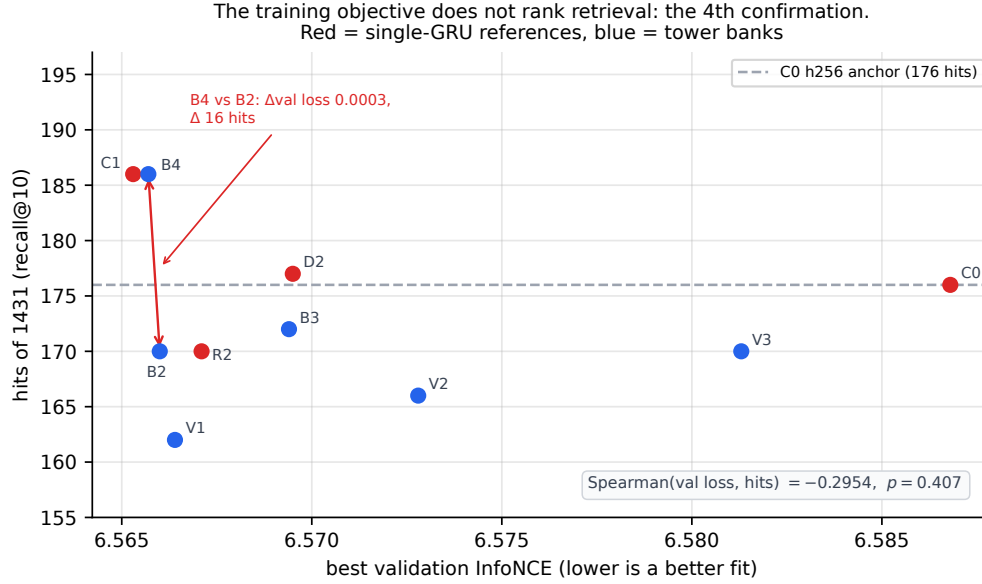
Figura 36: El objetivo de entrenamiento no ordena la recuperación: cuarta confirmación, y su instancia más nítida hasta ahora. Diez ramas del lote de bancos de torres: mejor InfoNCE de validación frente a aciertos de 1431. Spearman = -0,2954 , p = 0,407 . B4 y B2 distan 0,0003 en pérdida de validación y 16 aciertos; C0, el peor ajuste del lote, supera a seis de los ocho bancos. Todas las ramas pararon temprano (época 14 siete veces, luego 21 y 24 dos veces), así que el recall de ninguna rama es una cota inferior impuesta por el techo de épocas.
