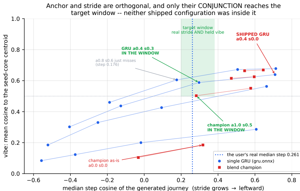
Figura 19: Los dos controles en tiempo de recuperación son ortogonales, y solo su conjunción alcanza la ventana objetivo (sombreada: paso mediano \in [0,20,0,38] y vibe \geq 0,50 ). Cada línea une un ancla fija a medida que crece la zancada, lo que mueve el viaje hacia la izquierda (pasos más grandes) mientras el vibe decae despacio — así que el compromiso es real pero suave. Ninguna configuración despachada está dentro de la ventana: la GRU con a = 0,4 , s = 0 sostiene un vibe de 0,639 pero camina a 0,709, y el campeón tal como se despliega camina a 0,318 con un vibe de 0,185. 20 sesiones held-out \times 20 pasos, cap 1 ( tools/walk_frontier.py ).
