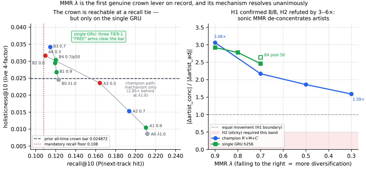
Figura 14: Izquierda: la frontera de \lambda en el plano recall \times corona. Cada motor traza un camino a medida que \lambda baja desde 1,0; el color es el nivel pre-registrado (verde NIVEL-1 GRATIS, azul NIVEL-2 CON PRECIO, rojo NIVEL-3 RECHAZADA, gris control). Tres ramas de la GRU única superan la barra histórica de corona 0,024872 con un recall cuyo IC pareado abarca cero — el primer movimiento de corona genuinamente gratuito del registro. El camino del campeón alcanza un H comparable solo tras pagar recall que el IC ve, y sus dos mejores puntos de H quedan rechazados como degenerados. Derecha: la pregunta de mecanismo. H1 exigía |\Delta \text{artist\_conc}| \geq |\Delta \text{artist\_adj}| ; H2 exigía la razón por debajo de 0,5 (zona sombreada). Medida en 1,59 a 3,06 en 8 de 8 ramas, así que H2 queda refutada por un factor de 3 a 6 en la dirección contraria — y la razón se encoge monótonamente al bajar \lambda , es decir, la des-concentración fácil se compra primero y el mecanismo se satura.
