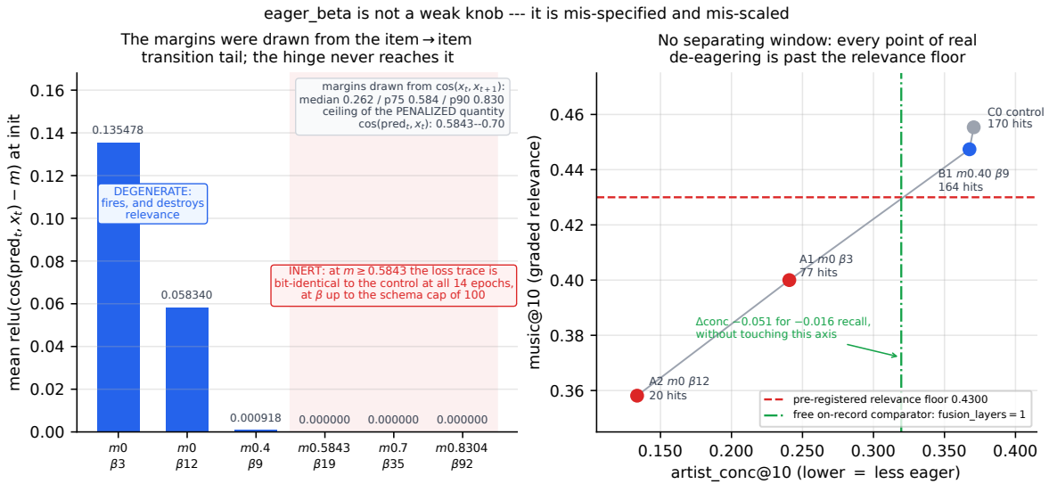
Figura 16: Izquierda: el resultado central de la campaña. La penalización realizada del hinge en la inicialización, reconstruida a partir de la inflación de la pérdida en la época 1 con inicialización compartida (semilla idéntica, así que inicialización y orden de lotes idénticos). Los márgenes se calibraron desde el coseno de transición ítem → ítem (mediana 0,262, p75 0,584, p90 0,830), pero la penalización actúa sobre predicción → actual , cuyo techo a lo largo del entrenamiento se sitúa entre 0,5843 y 0,70: con m \geq 0,5843 la cantidad penalizada nunca entra en el soporte del hinge y la traza de pérdida es idéntica bit a bit a la del control en las 14 épocas, con \beta hasta el tope del esquema. Derecha: donde el mando sí dispara, eagerness y relevancia son el mismo mecanismo. Empujar la predicción lejos del latente de la pista actual la empuja también fuera de la región donde vive la verdadera pista siguiente, así que no hay ventana entre un des-eagering real y romper el umbral de relevancia. La línea de trazo y punto marca el comparador gratuito ya registrado que ninguna rama de aquí igualó dentro del umbral.
