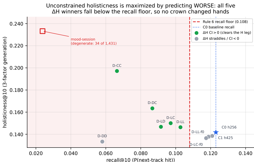
Figura 10: Por qué la regla de corona necesita un piso de recall duro. A lo largo de las diez ramas, \text{holisticness@10} corre casi exactamente al revés que Recall@10: las cinco ramas que superan el tramo de \Delta H con IC por encima de cero (verde) son las cinco más alejadas por debajo de la línea base en recall exacto, y las cinco caen fuera del piso de \pm 0,015 (sombreado). El cuadrado hueco es el modelo incumbente mood-session que motivó el piso: la mayor holística del registro con 34 de 1431 pistas siguientes correctas. Los valores de H son de la generación de 3 factores (Sección 18).
