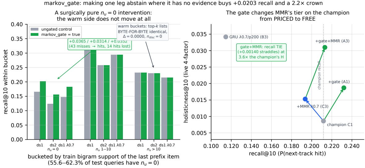
Figura 15: Izquierda: la descomposición por bucket sobre los tres pares control/rama (ds1 canónica, ds2 la segunda partición con 64% de fríos, ds1 \lambda 0.7 el mismo par canónico bajo un re-ordenamiento MMR). El efecto entero se sitúa en el bucket de soporte cero; en ambos buckets cálidos las listas top- k de las ramas son idénticas byte a byte, y por eso un peso global de rama no puede expresar demostrablemente esta intervención. Derecha: el mismo resultado en el plano recall \times corona. MMR por sí solo (azul) es una palanca con precio en el campeón: compra corona y pierde recall con el IC bajo cero. La compuerta (verde) compra ambos . Compuestas, compuerta+MMR aterriza en el recall del campeón ( \Delta +0,00140 , abarcando) con 3,6× su holistcness, así que la compuerta cambia el nivel de MMR en el campeón de CON PRECIO a GRATIS.
