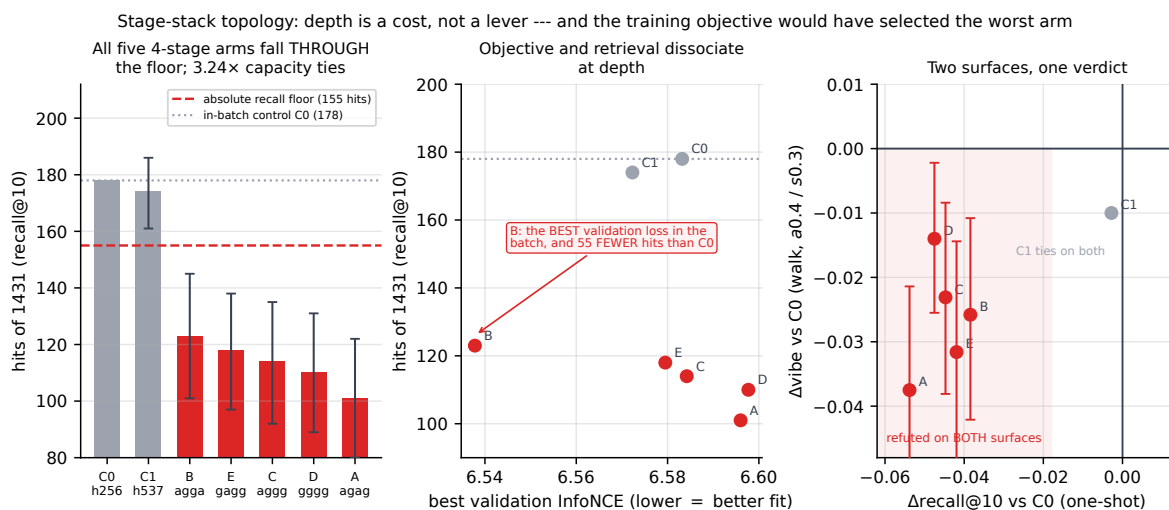
Figura 21: Izquierda: las cinco ramas de 4 etapas caen por debajo del umbral absoluto obligatorio de recall, mientras el control de capacidad 3,24× empata con el ancla — así que el daño es la profundidad, no la capacidad. Las barras de error son el IC bootstrap pareado contra el control del mismo lote, proyectado sobre la escala de aciertos. Centro: el número más interesante de la campaña. La rama B alcanza la mejor pérdida InfoNCE de validación del lote y recupera 55 aciertos menos que el control: el objetivo que entrena toda la familia y la calidad de recuperación del top-10 se desacoplan en profundidad, así que cualquier búsqueda de arquitectura que seleccione por pérdida de validación elegiría la rama equivocada. Derecha: el cierre en dos superficies. La lectura de caminata en la celda primaria igualada refuta las mismas cinco ramas que refuta la superficie de un solo disparo; el control de capacidad empata en ambas. El eje no falla meramente en cerrarse en una superficie: se cierra en dos.
