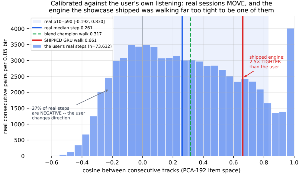
Figura 17: El argumento central de esta sección, en una figura. Los 73 632 cosenos de transición consecutiva del propio usuario (espacio de ítems PCA-192, solo sesiones de entrenamiento) forman una distribución ancha : mediana 0,261, p10–p90 [−0,192, 0,830], 27,0 % de pasos negativos. El motor que el showcase despachó camina con un paso mediano de 0,661 — unas 2,5× más ceñido que la persona a la que imita — y ninguna métrica de un solo disparo podía verlo, porque holisticness@10 puntúa un top-10 y su mood_coh se ancla a un centroide de prefijo que crece con la caminata. El campeón de blend (0,317) iguala el paso real pero no logra sostener un vibe . Recuentos por bin transcritos del bloque de calibración de tools/walk_eval.py .
