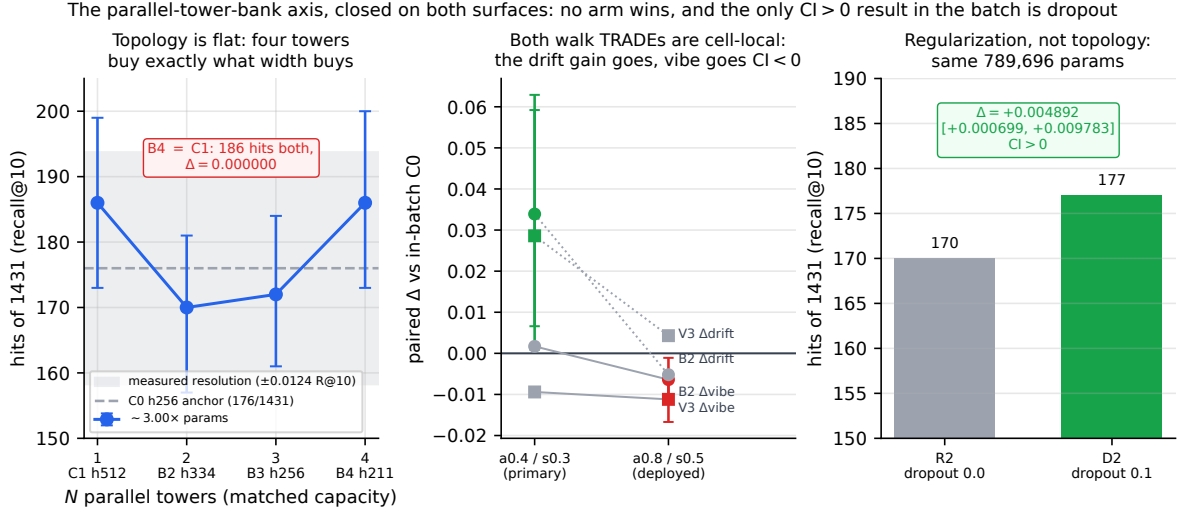
Figura 22: El eje de bancos de torres paralelas, cerrado en ambas superficies. Izquierda: el eje N a capacidad igualada ( \sim 3,00\times la línea base h256). Las barras de error son el IC bootstrap pareado contra C0 proyectado a la escala de aciertos; la banda gris es la resolución medida de la partición ( \pm 0,0124 recall@10 = \pm 17,7 aciertos, Figura 13), y todas las ramas caen dentro. Cuatro torres h211 (B4) y una GRU h512 (C1) devuelven los mismos 186 aciertos, con \Delta pareado 0,000000. Centro: las dos ramas que lograron un TRADE de caminata en la celda primaria voltean en la celda desplegada: la ganancia de deriva que compró el TRADE decae hasta cruzar el cero mientras el vibe se va por debajo. Los marcadores grises son estimaciones puntuales cuyo IC cruza el cero (el informe fuente solo cita límites para los intervalos que no lo cruzan). Derecha: el único resultado positivo de la campaña, y no es sobre topología — con parámetros idénticos byte a byte (789 696 en ambos, model.pt de 3 162 277 bytes en ambos) el dropout 0,1 supera al dropout 0,0, con el IC por encima de cero.
