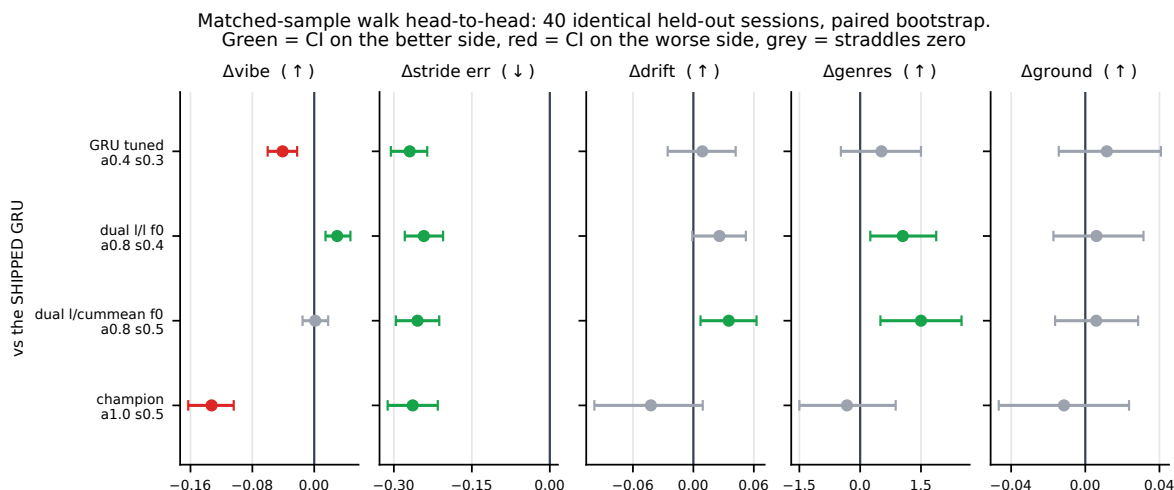
Figura 20: El cara a cara de muestra emparejada, un panel por métrica en su propia escala — deliberadamente sin eje doble, que insinuaría una comparabilidad que estas cinco cantidades no tienen. El verde es un IC enteramente en el lado bueno de la métrica, el rojo enteramente en el lado malo, el gris cruza el cero. Todas las ramas compran la zancada real; solo las ramas de torre doble la compran sin pagar vibe, y ground cruza el cero en todas las ramas.
