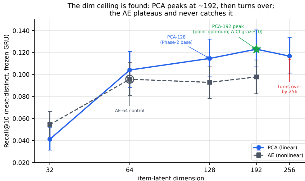
Figura 2: Se encuentra el techo de dimensión. Extendiendo el barrido de compresión de la Figura 1 a PCA-192/256 y AE-192, la curva PCA (azul) hace pico en ~192 (R@10 0,123) y se revierte hacia 256, mientras que el AE (gris) se estanca plano en \sim 0.09 – 0.10 y nunca lo alcanza — la brecha \text{PCA} \geq \text{AE} es máxima en 192. PCA-192 es el óptimo puntual (estrella verde) pero su \Delta pareado sobre PCA-128 roza cero, así que PCA-128 se mantiene como la base individual de la Fase 2. Las barras de error son IC bootstrap al 95 % sobre las 1431 sesiones de prueba.
