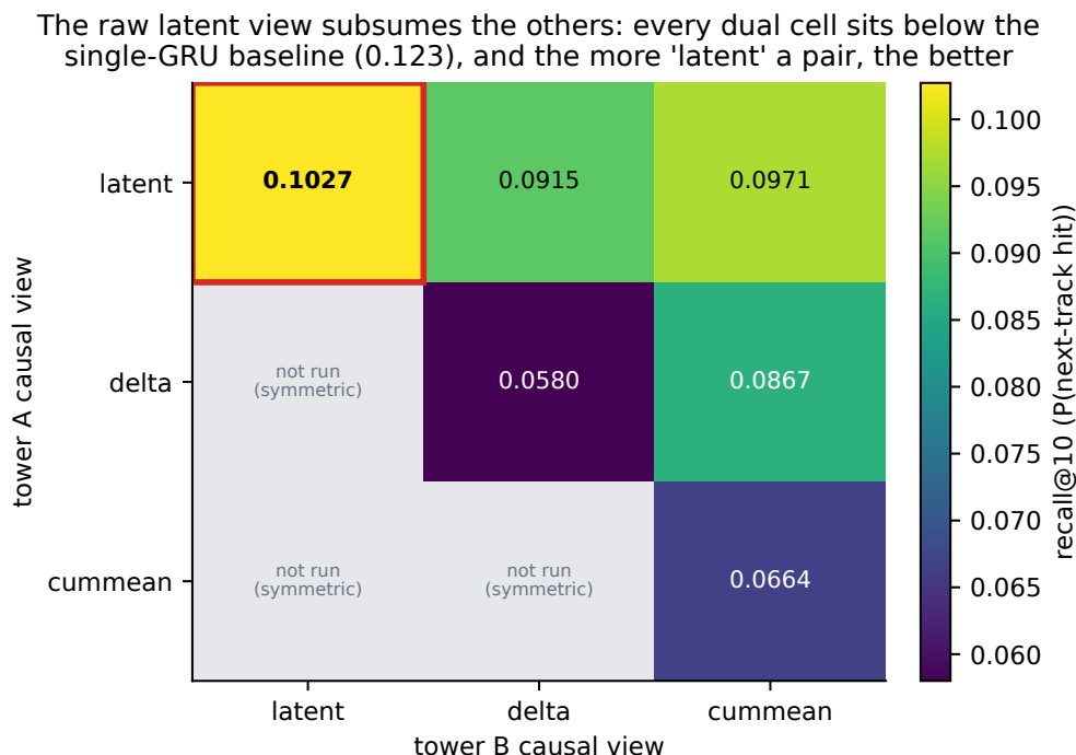
Figura 9: La matriz completa de emparejamiento de vistas con fusion_layers = 1 , una ejecución por celda. Toda celda dual queda por debajo de la línea base de GRU única (0,12299), y el orden es monótono en cuánta vista latent cruda contiene el par: ambas-latent es la mejor, ambas-delta la peor. El triángulo inferior nunca se ejecutó (el emparejamiento es simétrico por construcción) y se enmascara en gris en lugar de reflejarse, de modo que la escala de color refleja solo celdas medidas. El gradiente es el hallazgo: una torre recurrente sobre latentes crudos ya calcula lo que delta y cummean hacen explícito.
