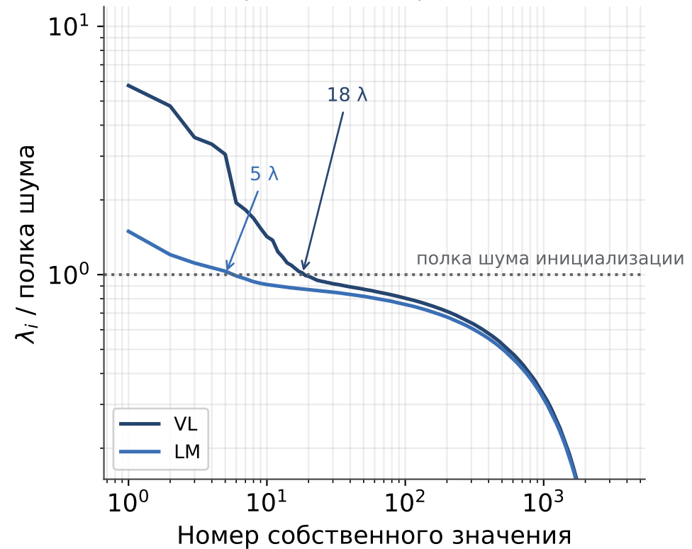
в) веса направлений метрики ( m = 3584 )
