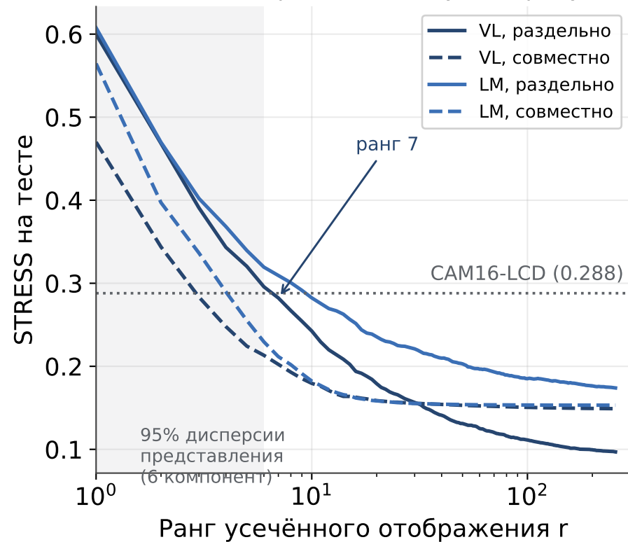
а) сколько направлений несут метрику
