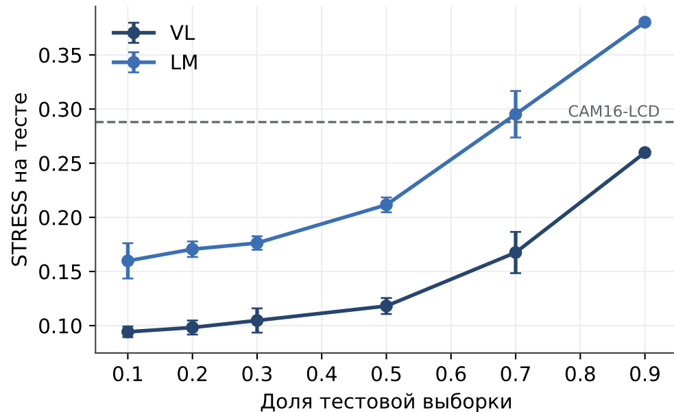
Манселл (сплит по цветам, group-k)
