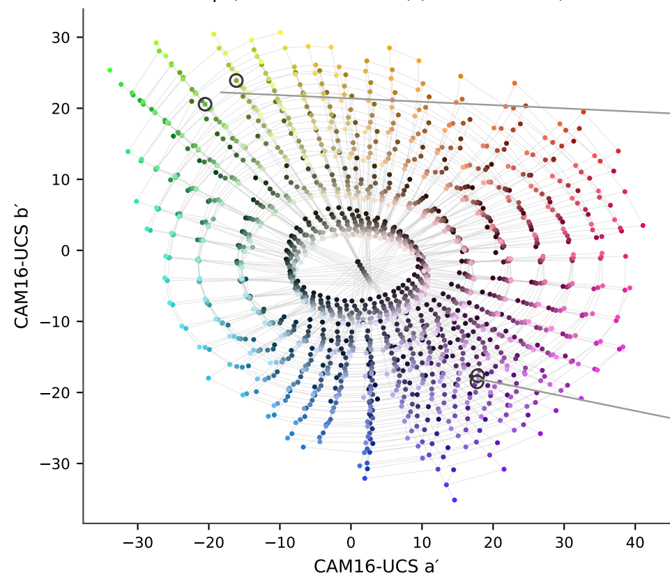
Цветовые центры Манселла и единичные перцептивные шаги (цепочки H/C/V)
