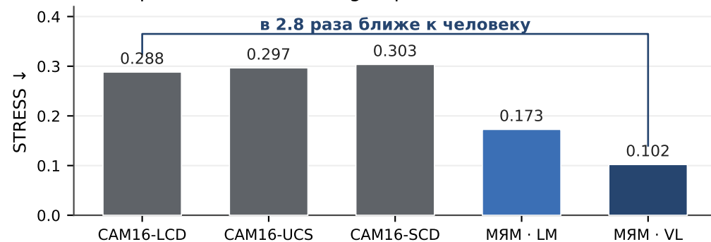
Надпороговые · Манселл (group-k, те же цвета)
