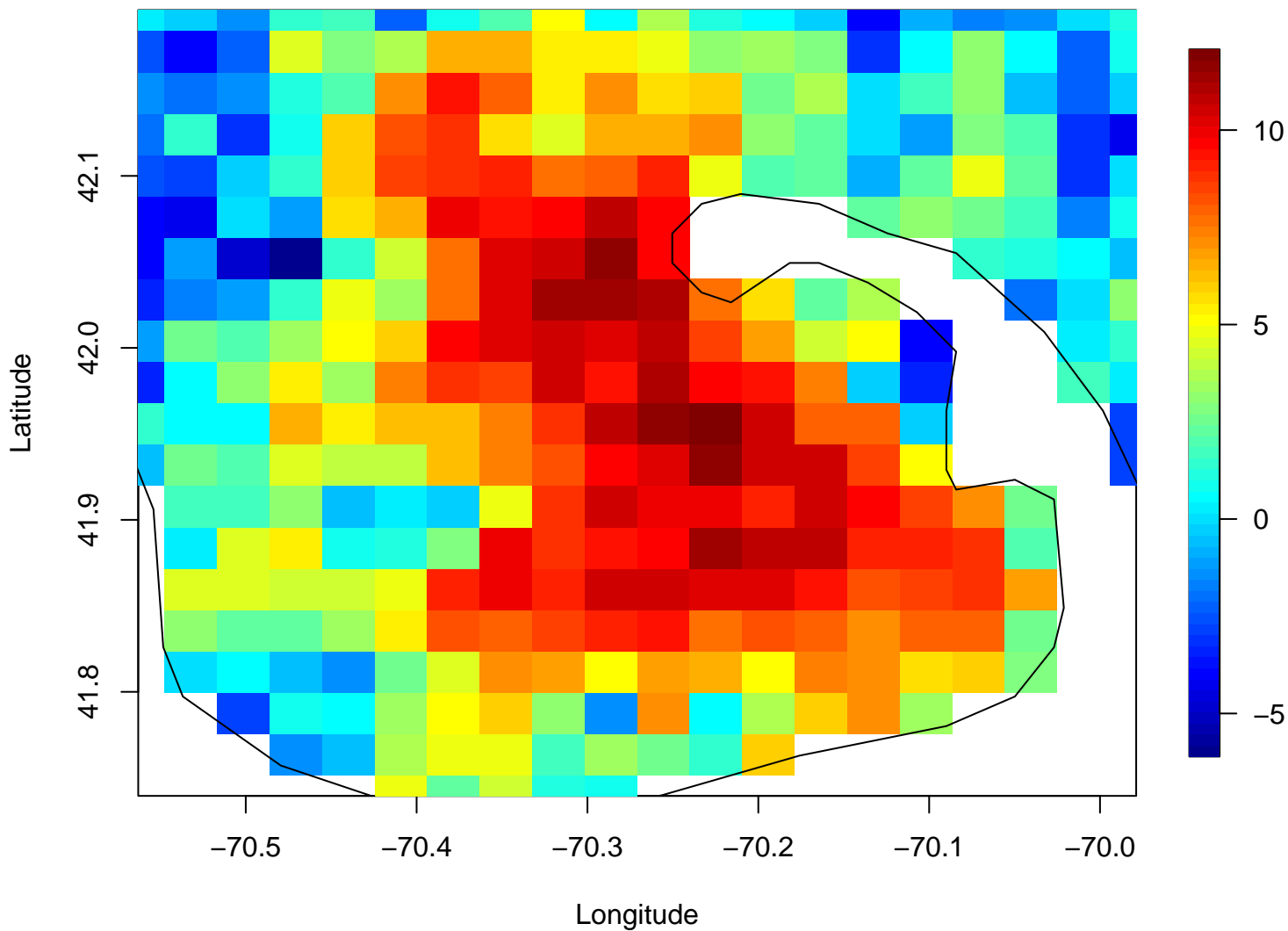
Fused Data Posterior Intensity Surface
