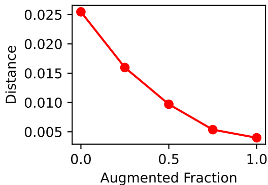
MMD Hausdorff
