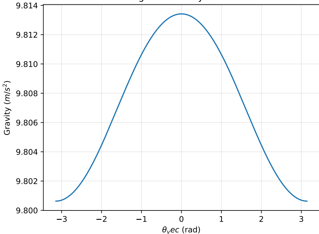
Somigliana Gravity Variation
