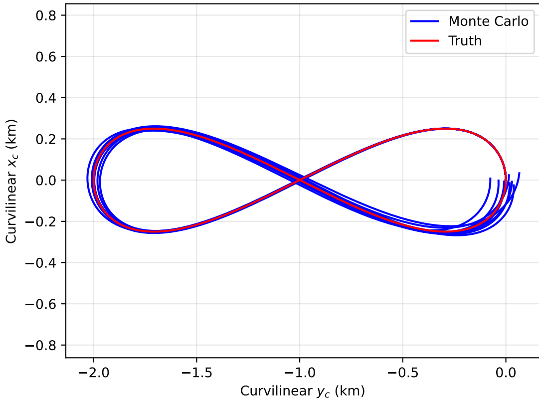
accel_x: Horizontal Trajectories
