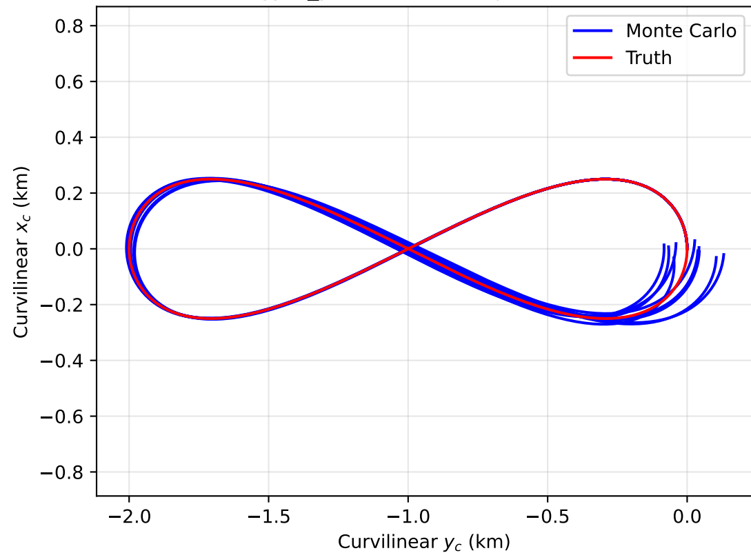
gyro_y: Horizontal Trajectories
