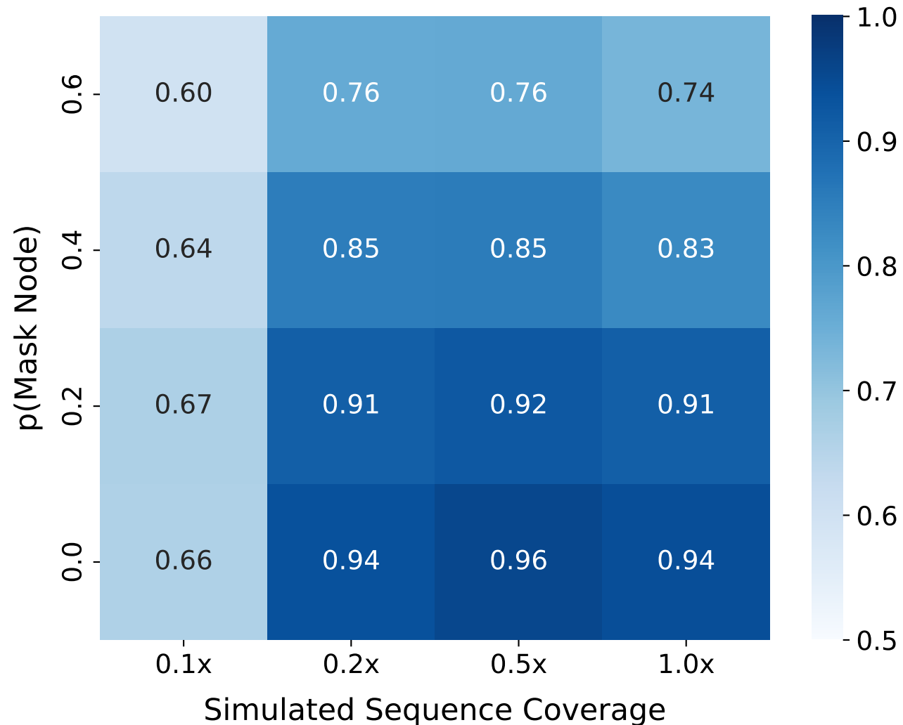
Relation F1 Scores
