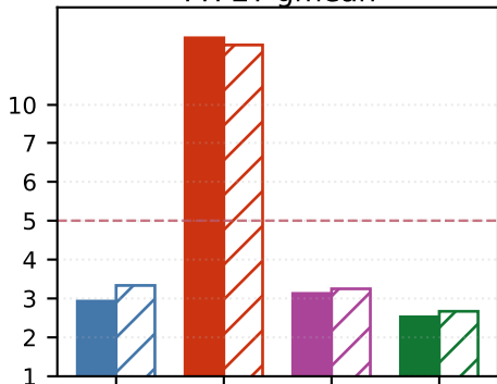
E2E gmean
