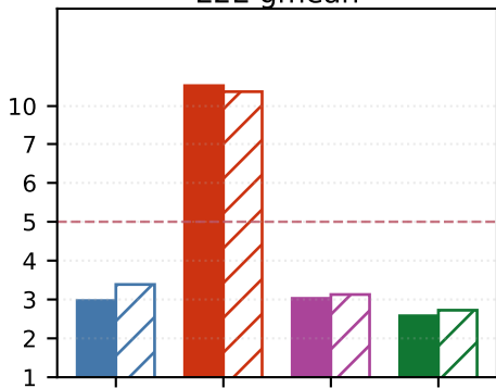
E2E gmean
