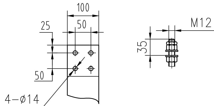
低压端子接线图
