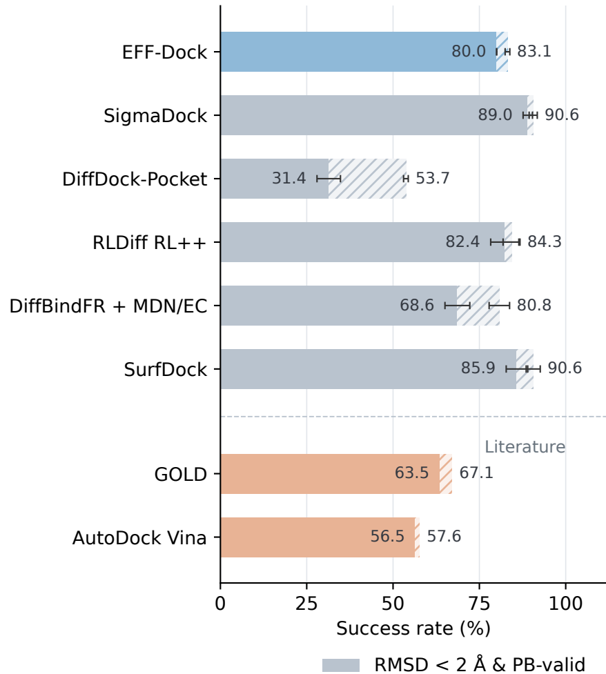
A Astex Diverse Set
