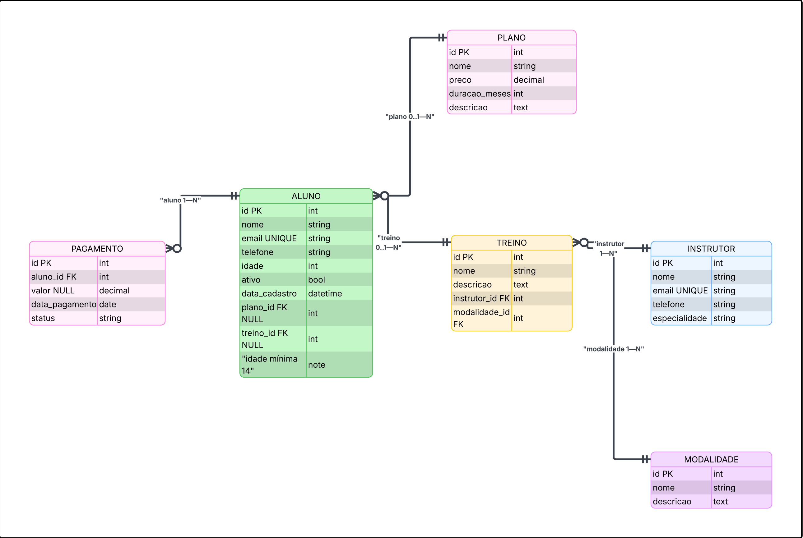
Diagrama ER - Academia
