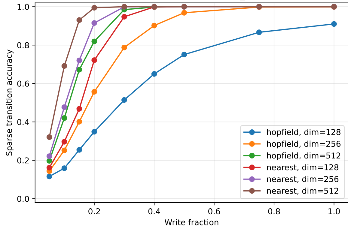
Sparse transitions (random_noise)
