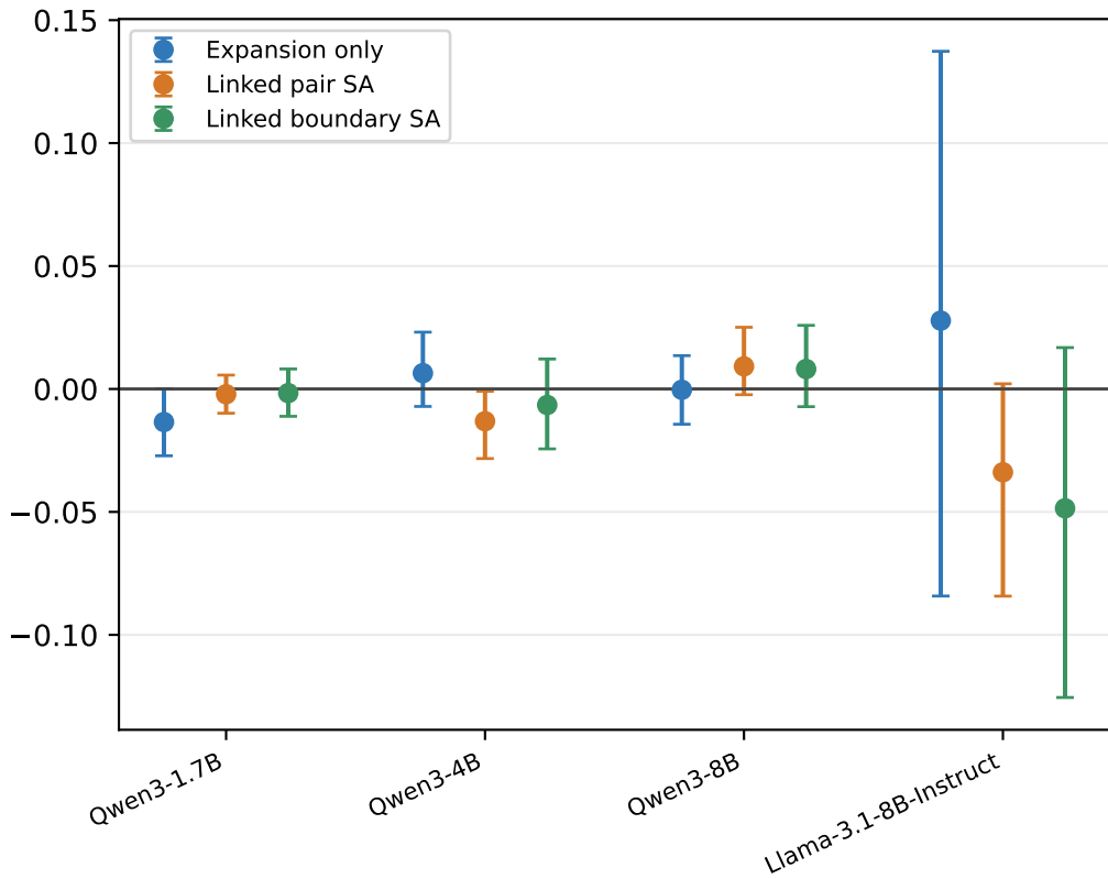
F1 delta vs independent PRA
