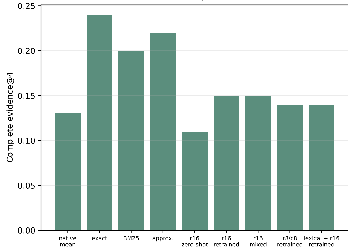
MuSiQue
