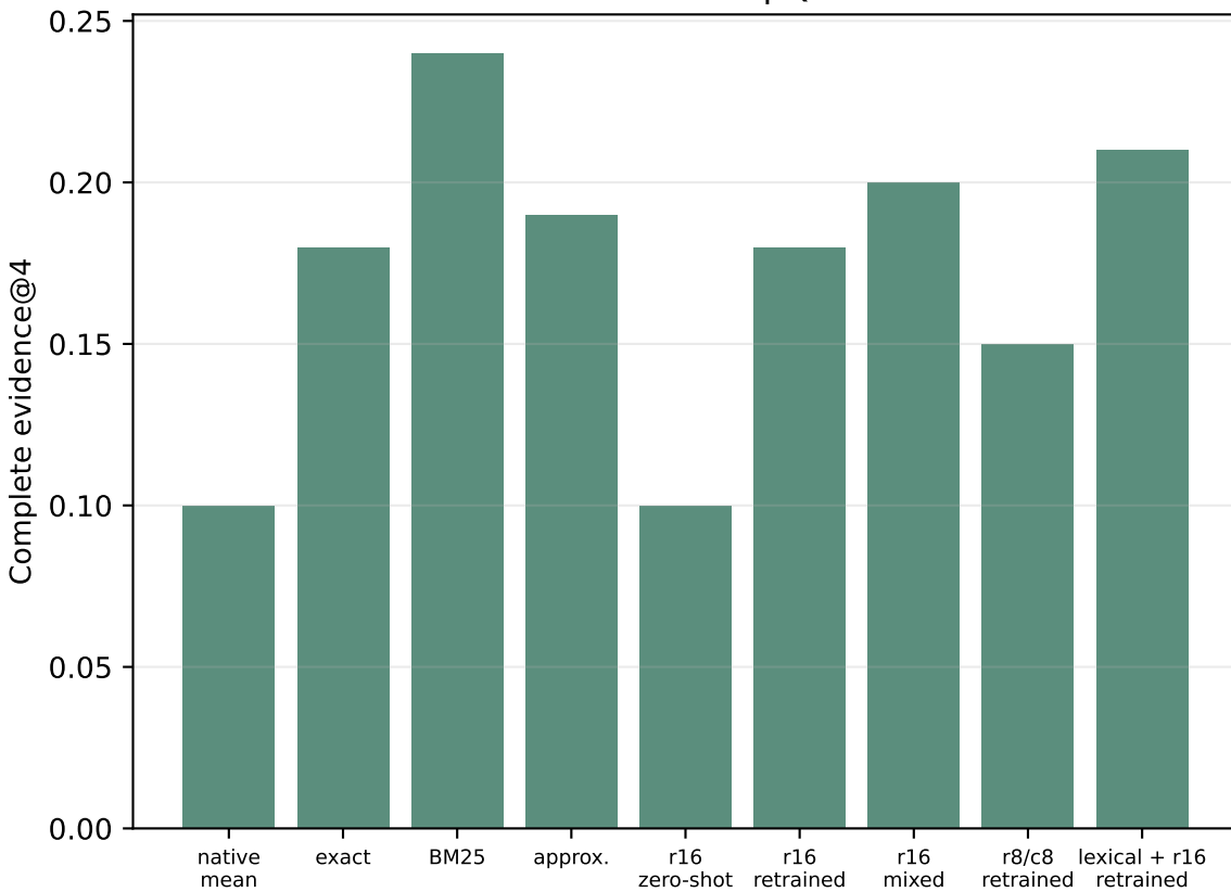
2WikiMultiHopQA
