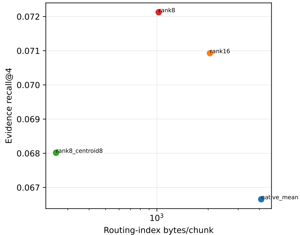
MuSiQue
