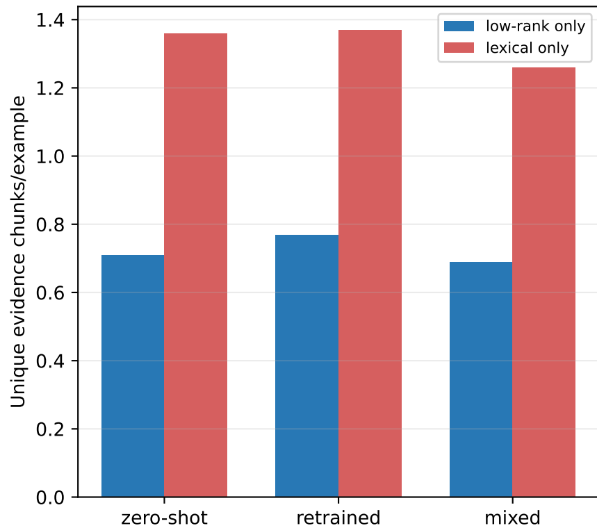
MuSiQue
