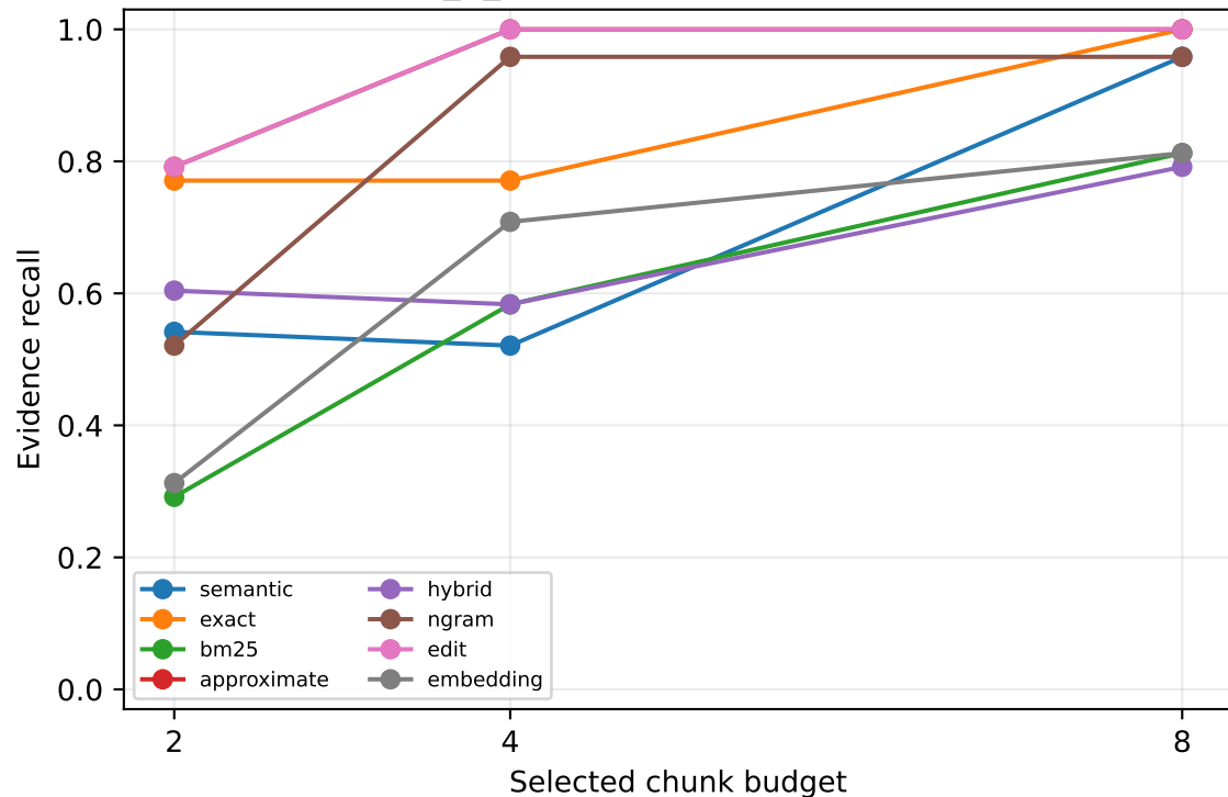
smollm2_135m / qasper (32-token chunks)
