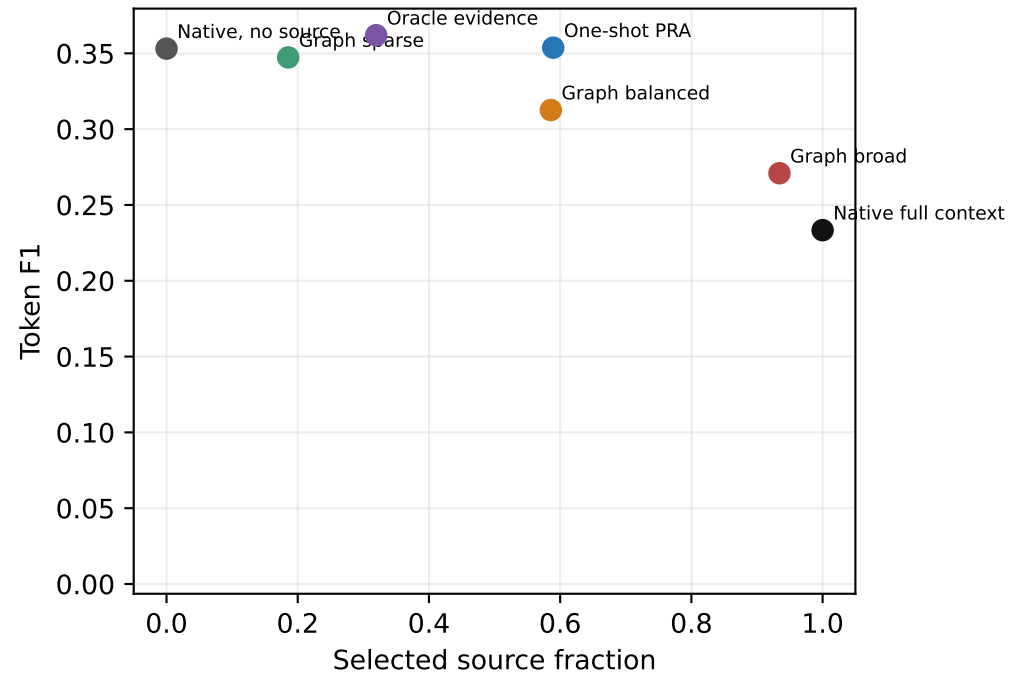
2Wiki
