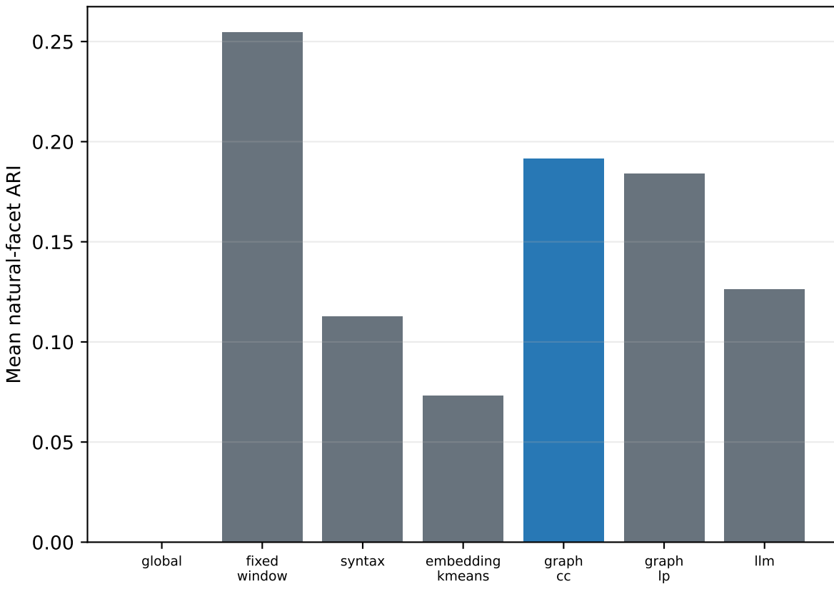
Qwen3-0.6B
